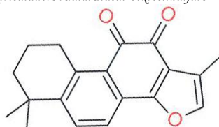
\text{C}_{19}\text{H}_{18}\text{O}_3 molekula szerkezete
