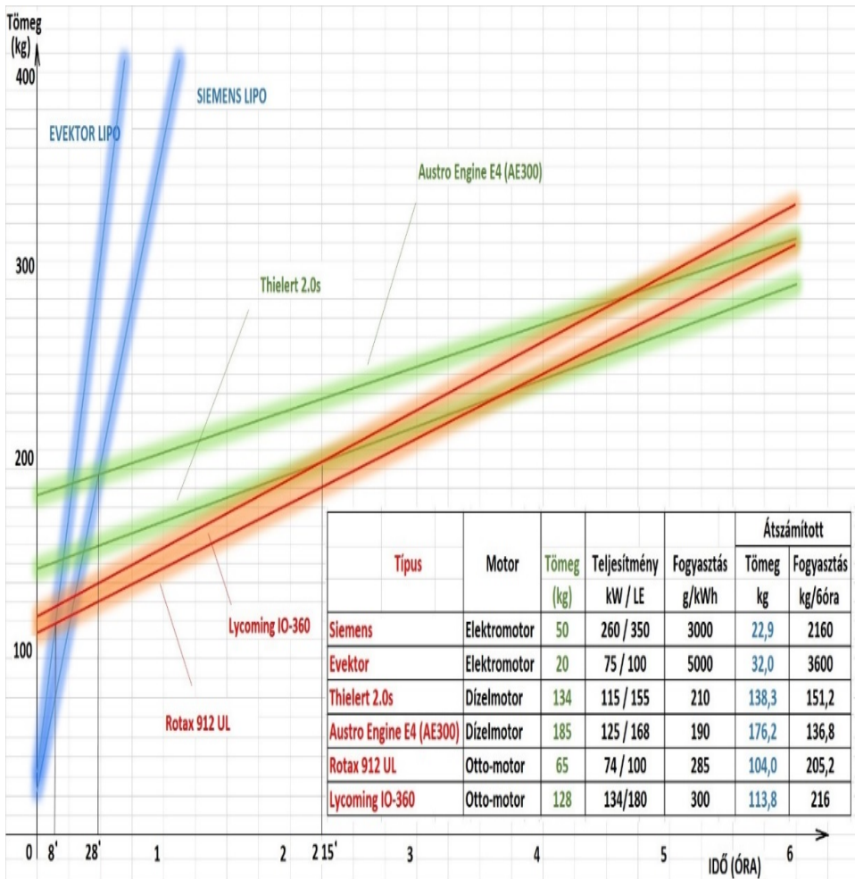
1. ábra. A benzin-, dízel- és az elektromos motorok adott repülési időhöz szükséges tömegdiagramja. 5
