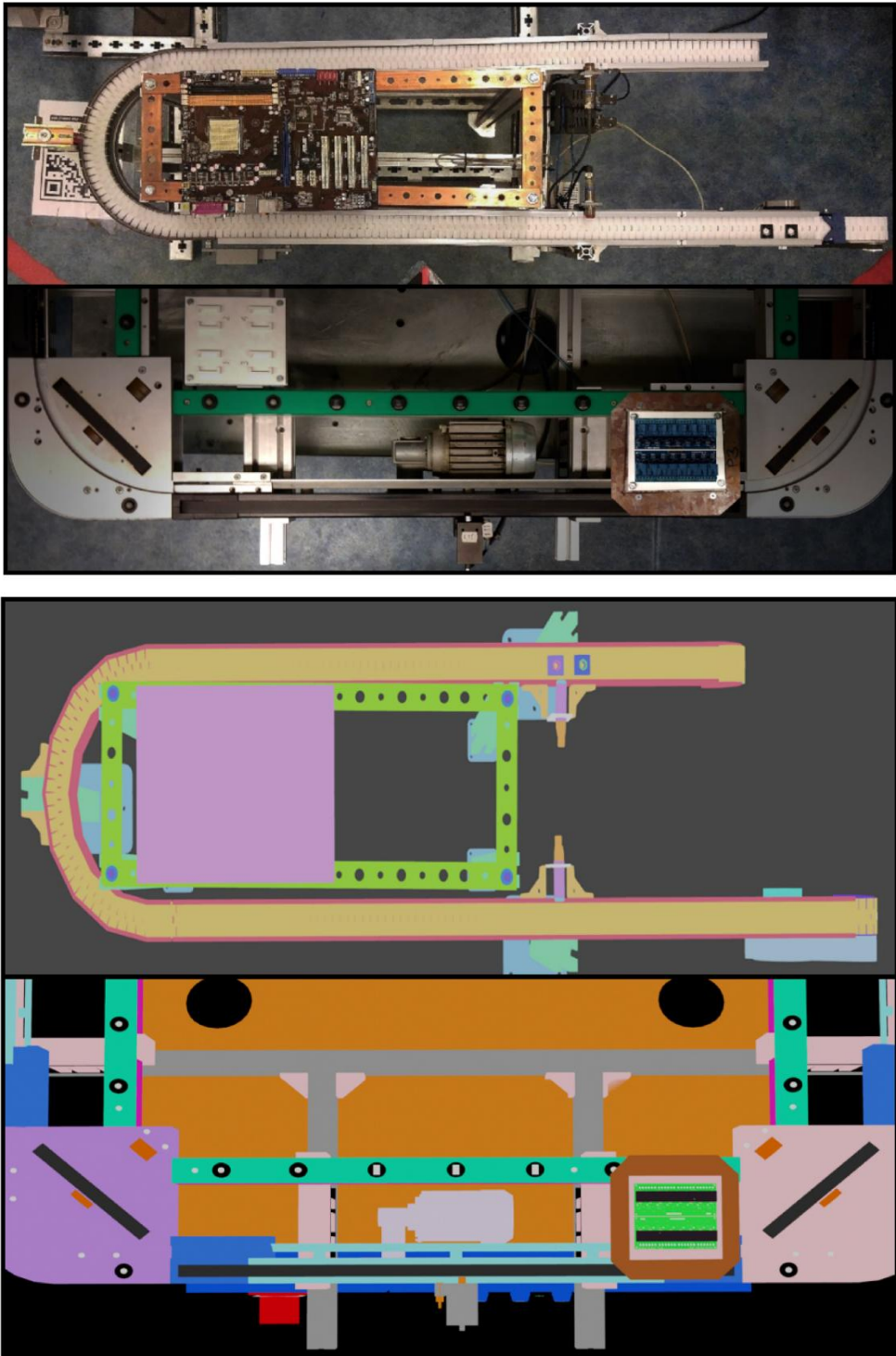
4. számú ábra. A Flexlink XK és PARO QE szállítószalag (-konveor) és a 3D CAD-alapú képkötés alapján előállt képe
