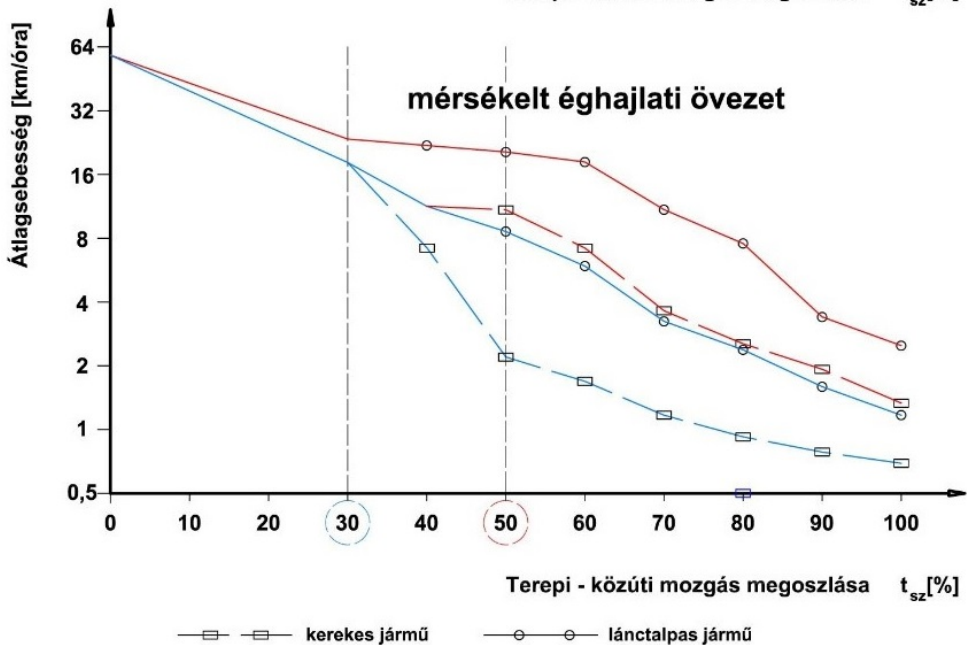
6. számú ábra. Lánctalpas és kerekes páncélozott harcjárművek átlagsebességének alakulása a terepszázalék függvényében [7/3–45_3–52] (készítette a szerző)
