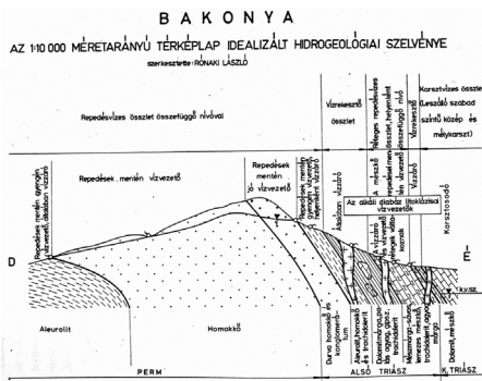
17. Kép: Bakonya É-D irányú földtani szelvénye.
