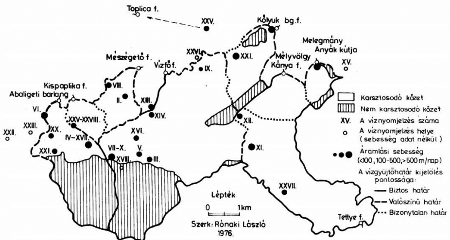
15. Kép: Víznyomjelzések, és értelmezésük. (1976)
