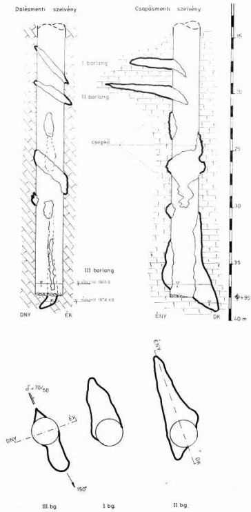
16. Kép: A siklói barlangok szelvényvázatai. (1978)
