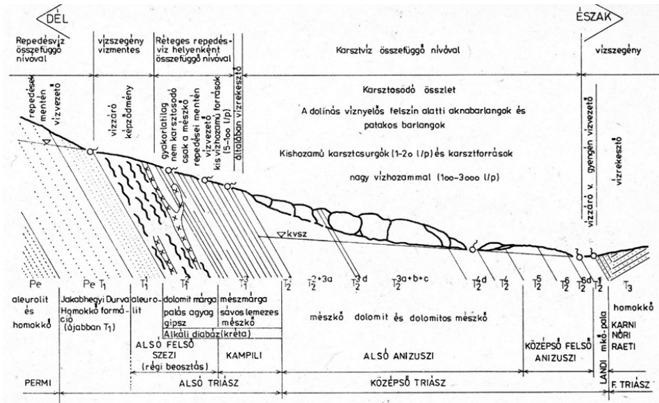
21. Kép: A Ny-Mecsek idealizált földtani-hidrogeológiai szelvénye.
