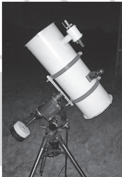
A 260/4100-as, Csatlós Géza által épített Nasmyth-távcső 1998-ban, eredeti mechanikáján (balra), és 2022-ben, az észlelőréten (jobbra)
