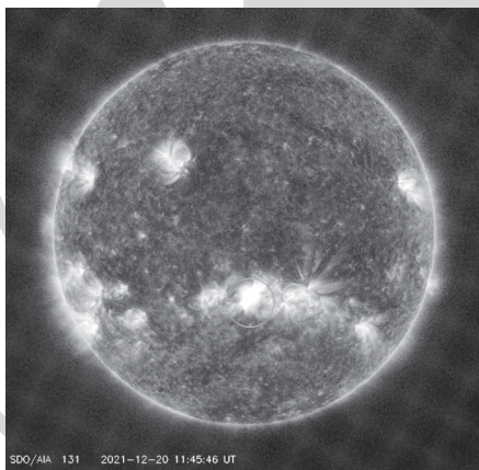
SDO/AIA 131 2021-12-20 11:45:46 UT
