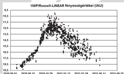
A 156P/Russell–LINEAR fénymenete az IAU fényességtételei alapján
