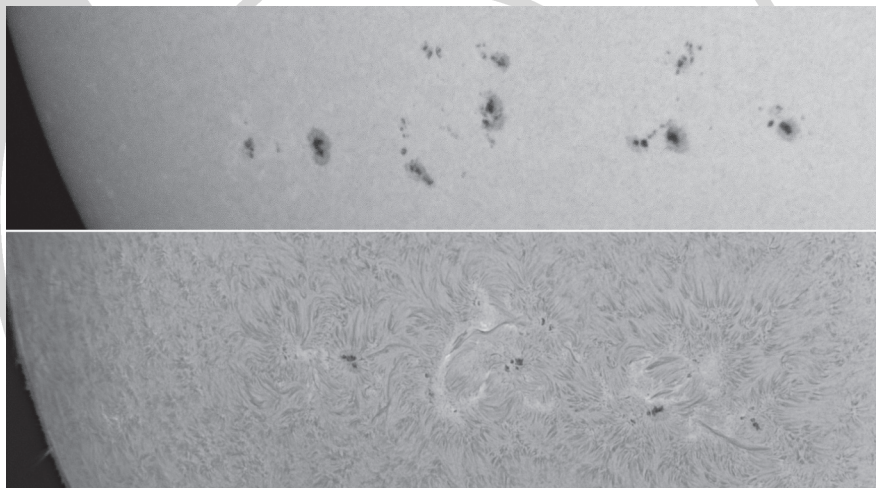
Központi csillagunk aktív területekben gazdag délkeleti része 2021. december 17-én fehér fényben (fent) és H-alfa tartományban (lent) Dézsi Attila felvételein
