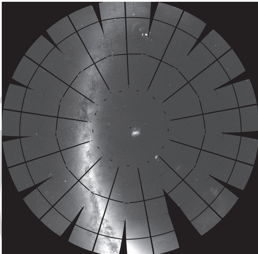
A déli égbolt a TESS szemén keresztül. A Tejút sávja mellett a Nagy Magellán-felhő (középen) és az Orion-köd (felül) is egyértelműen kivehető. A kép 13 szektor 208 felvételének felhasználásával készült (NASA/MIT/TESS)
