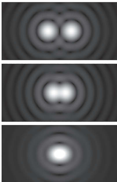
A legfelső kép mutatja a jól elkülönülő párokat, míg középen láthatjuk a Rayleigh határon lévő, halvány réssel bontott kettőscsillagok tipikus képét. A legalsó kép az adott műszerrel már fel nem bontható objektumok látványát modellezi (wikipedia.org)
