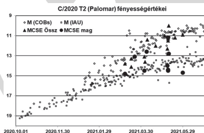
A C/2020 T2 (Palomar) fényességváltozása az IAU, a COBs és a hazai adatok alapján
