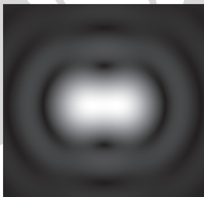
A szinte teljesen összeolvadó csillagokat észlelve is felfedezhetjük azok kettősségét (wikipedia.org)
