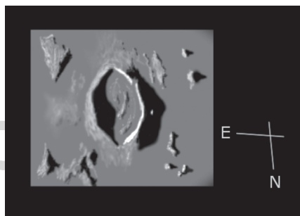
A Hansteen-kráter a Mons Hansteennal Földvári István Zoltán digitális rajzán. Észlelőnk ezt a szép rajzot 2019. február 16-án készítette a 70/500-as refraktorával, 100x-os nagyítást használva
