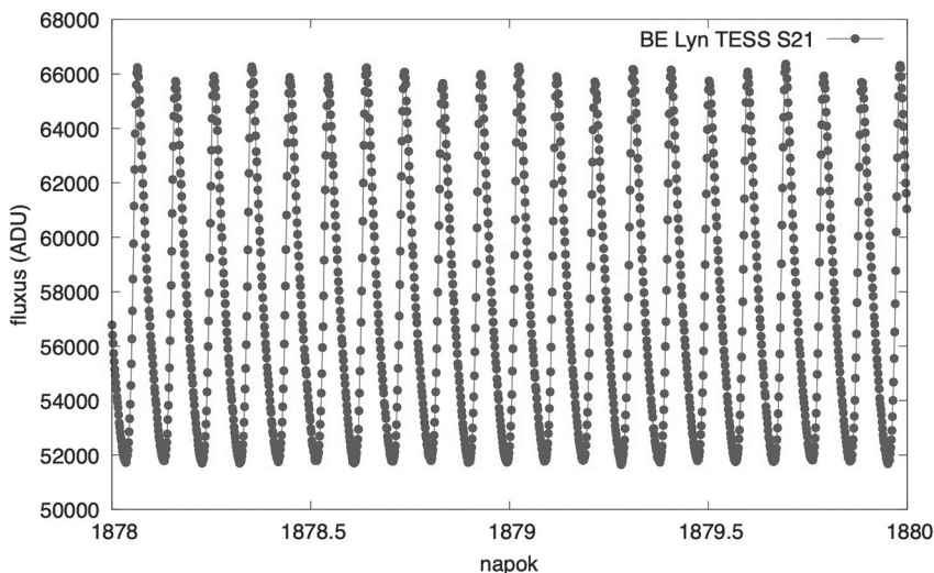
Két napnyi folyamatos TESS-fénygörbe a BE Lyn-ről. Ránézésre feltűnő, hogy míg a minimumfényességek jó közelítéssel állandóak, a maximumok ciklusról ciklusra kicsit ingadoznak. Részletes elemzés igazolja, hogy ezt nem a mintavételezés okozza
