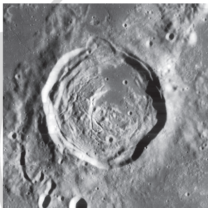
A Hansteen-kráter a Lunar Orbiter IV felvételén
