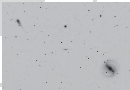
Sebestyén Attila 2021. május 8-án fotózta a C/2020 R4 (ATLAS) üstököst az NGC 4314 galaxis közelében. (150/750 T + ASI 174 MM; Gain 200; 60x30 s)
