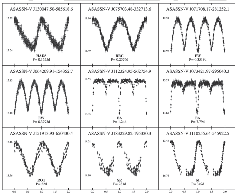
Periodikus változócsillagok az ASAS-SN adataiban (ábra: ASAS-SN weblap)
