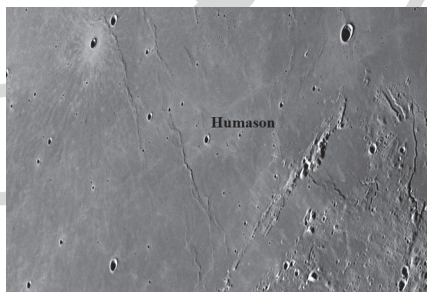
A 4 kilométer átmérőjű Humason-kráter Csabai István 2018. szeptember 5-én készült felvételén (C-14-es Schmidt-Cassegrain, Basler scA2040-120um IMX 252 kamera)
