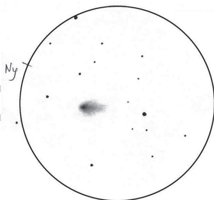
Sánta Gábor rajza a 156P/Russell–LINEAR üstökösről 2021. január 9-én készült. 355/1650 T; 206x-os nagyítás, a látómező 21 ívperc átmérőjű
