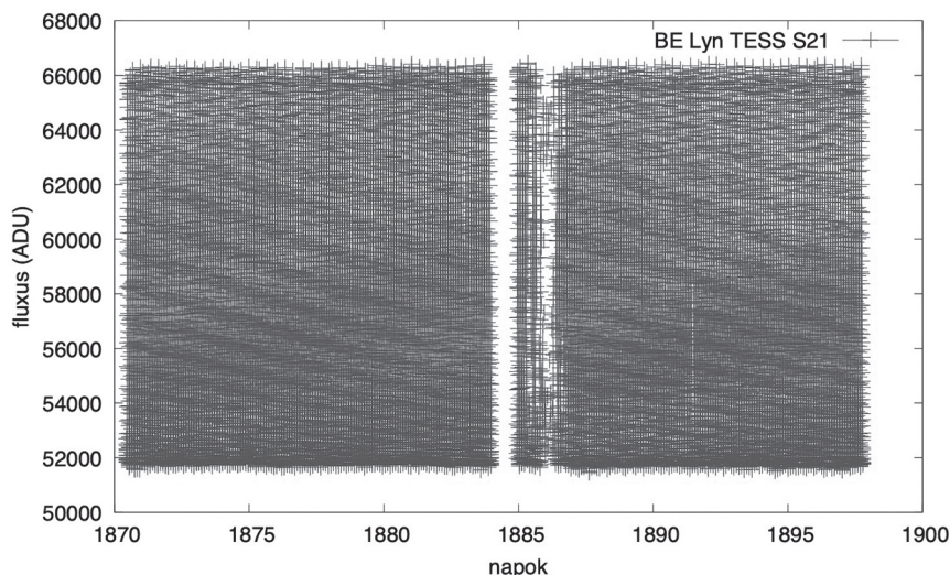
A BE Lyn TESS-adatai a 21-es szektorban. A vízszintes tengelyen az idő napban, a függőleges tengelyen a csillag fényessége fluxus egységekben (a nagyobb szám felel meg a fényesebb állapotnak)
