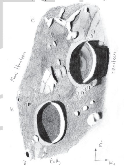
2022. január 14-én Görgei Zoltán ismét észlelte a kráterpárost a Mons Hansteenel együtt, a 90/1000-es refraktorral, 250x-es nagyítással, zenittükörrel
