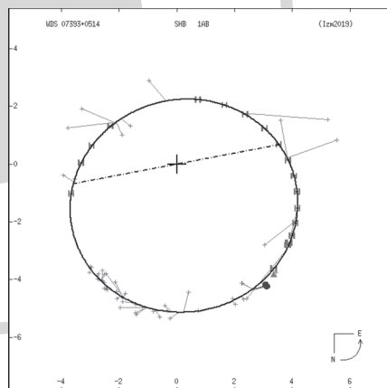
A Procyon pályája (www.astro.gsu.edu/wds/orb6)
