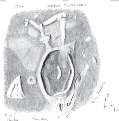
A Hansteen-kráter, a Rima Hansteen és a Mons Hansteen magas napállásnál, ahogyan a rovatvezető 2021. február 24-én látta (90/1000-es refraktor, 250x-es nagyítás, zenittükör)
