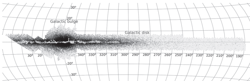
66 ezer OGLE-mira elhelyezkedése a Tejútrendszerben (Iwanek és munkatársai 2022)
