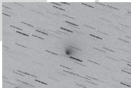
Sebestyén Attila a legyezőszerű csóvát mutató üstököszt 2021. február 15-én fotózta (150/750 T + ASI 174 MM; Gain 200; 20x120 s)
