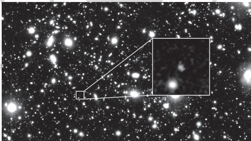
A legtávolabbi eddig ismert, HD1 jelű galaxis – az inzett közepén (Harikane et al.)
