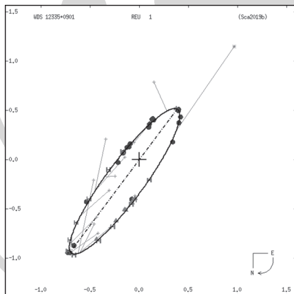
A Reu 1 pályája a pozíciószámítások alapján ( www.astro.gsu.edu/wds/orb6 )
