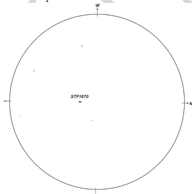
A Porrima 2021. június 4-én, 12 L, 111x: Lenyűgöző látványt nyújt. Két sárga csillag, melyek korongjai első pillantásra összeérnek, majd hosszabb szemlélés után nagyon keskeny réssel bomlanak (Szamosvári Zsolt)
