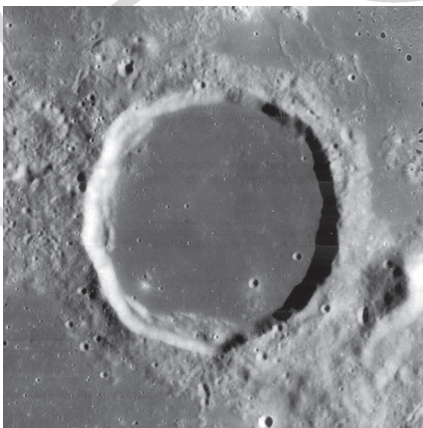
A Billy-kráter a Lunar Orbiter IV felvételén
