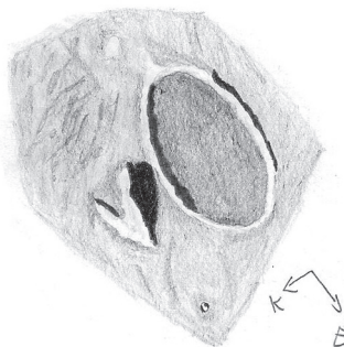
A Billy-kráter Erdei József bogyzslói tagtársunk rajzán. Ez a rajz egy 200/1000-es Newtonnal, 250x-es nagyítással készült
