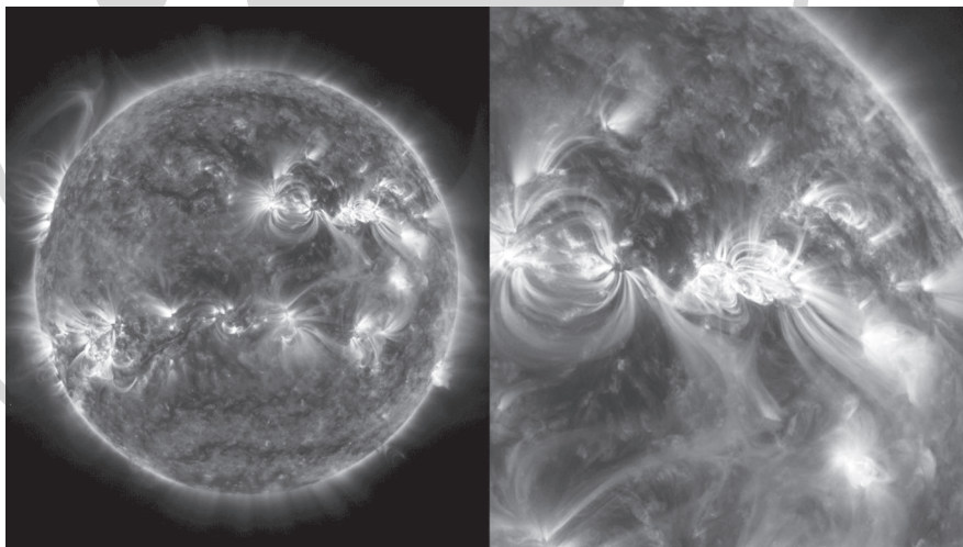
A NASA Solar Dynamics Observatory naptávcső-rendszerével lefényképezett fler (a kép kivágás közepén levő fényes folt). A 2022. március 30-án megjelent fler kifejlődése során az eredeti, az extrém ultraibolya tartományban készült képsorozaton kiválóan látható a napfelszínen végigsöprő lökéshullámfront is (kép: NASA SDO)
