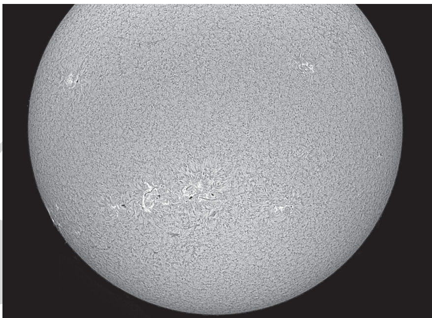
A Nap H-alfában, 2021. december 18-án
