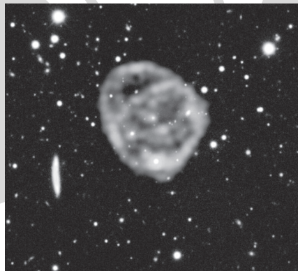
Az ORC-1 (Odd Radio Circle, Furcsa Rádiókör) felvétele. A MeerKAT rádiótávcső-hálózat adatait a Dark Energy Survey látható- és infravörös tartományban készült felvételeivel montírozták össze (J. English [U. Manitoba]/EMU/MeerKAT/DES/DOE/FNAL/DECam/CTIO/NOIRLab/NSF/AURA)
