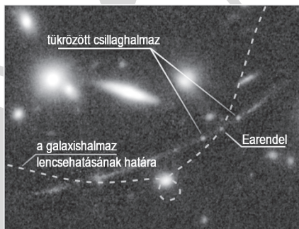
A közel 13 milliárd fényév távolságban levő, eddig ismert legtávolabbi csillag a Hubble-űrtávcső felvételén (NASA, ESA, Brian Welch [JHU], Dan Coe [STScI]; feldolgozás: NASA, ESA, Alyssa Pagan [STScI])
