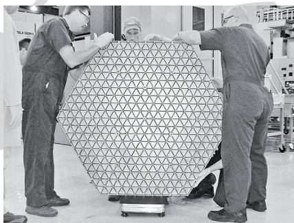
A James Webb-űrteleszkóp egyik berillium tükröszegmensének hátoldala készre munkálva. Jól látszanak a merevítők (kép: NASA)
