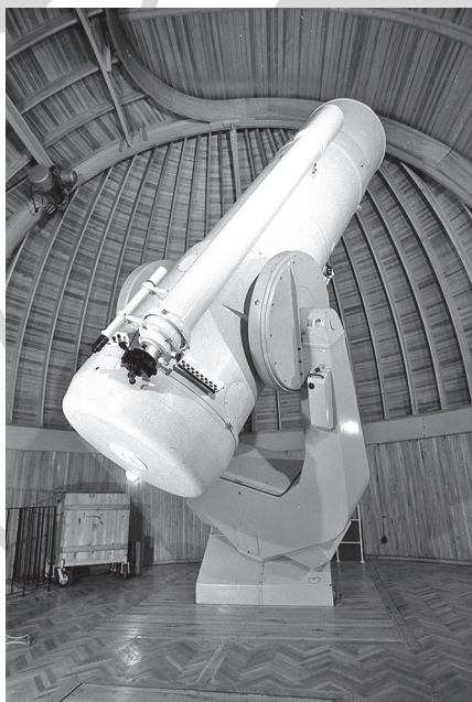
A piszkéstetői 60/90/180 cm-es Schmidt-távcső hazánk legeredményesebb felfedező műszere. Jelenleg egy olyan CCD-kamerával folynak az észlelések, amely 3x3 fokal látómezőt biztosít
