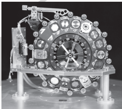
A James Webb-űrtávcső egyik főműszere, a MIRI (Max-Planck-Institut für Astronomie)
