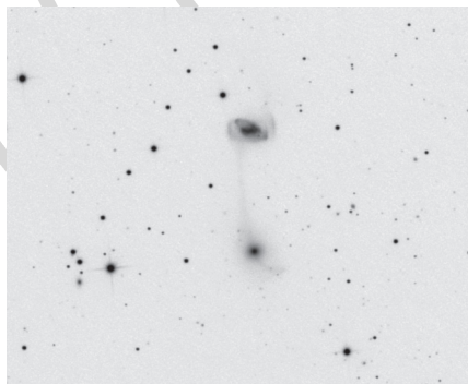
Az NGC 5216 és NGC 5218 párosa az Ursa Maiorban (Keenan's System) Sebestyén Attila felvételén (15 T, ASI178MM, 60x120 s)
