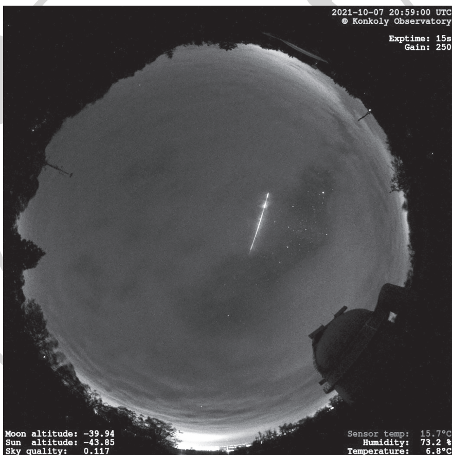
A 2021. október 7-én 20:59 UT-kor feltűnt tűzgömb Piskésetőről, az allsky kamerán (CSFK Csillagászati Intézet/Pál András)
