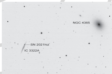
Az IC 3322A és a benne robbant SN 2021hiz Molnár Iván felvételén. A kép jobb szélén a fényes NGC 4365 látszik (28 SC, Canon EOS 600D, 27 \times 180 s, ISO 1600)
