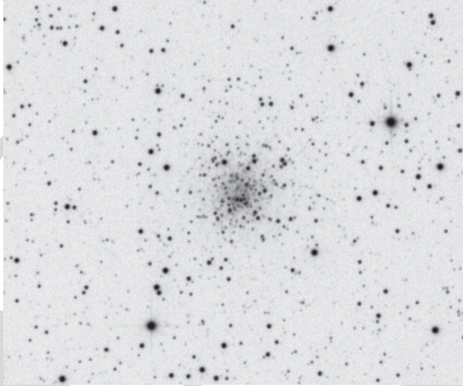
Sebestyén Attila felvétele az NGC 6426-ről (15 T, ASI174MM, 50x60 s)
