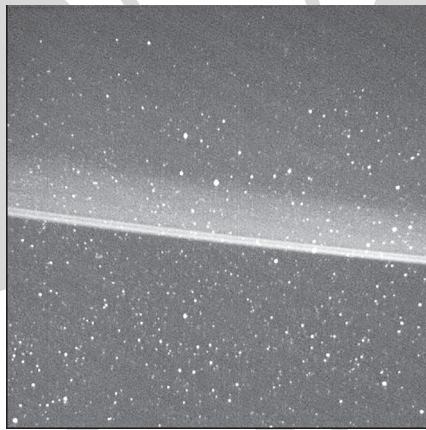
A Jupiter gyűrűje a Juno-űrszonda felvételén, 2021. szeptember 2-án. A legfényesebb rész a Metis és az Adrastea holdak pályáival áll kapcsolatban (NASA, JPL-Caltech)
