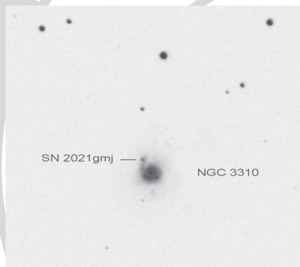
Az SN 2021gmj az NGC 3310-ben, Molnár Iván felvételén (28 SC, Canon EOS 600D, 3x180 s, ISO 800)
