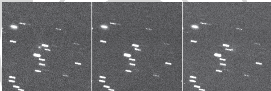
A C/2022 A1 (Sárneczky)-üstökös felfedezését eredményező január 2-ai felvételek. A tucatnyi képet négyesével, az üstökös mozgására adtam össze. Jól átható, hogy a felfedezést kis híján meghiúsította pár fényes háttércsillag, de szerencsére az első négy felvételen még tiszta égi háttér előtt mozgott a vándor
