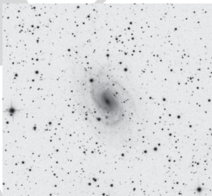
Az NGC 6384 GX Oph Gerák Ferenc fotóján (20 T, ASI533, 95 \times 180 s)
