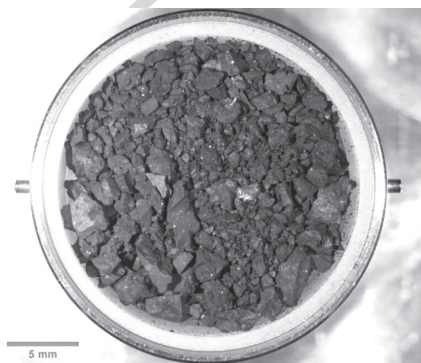
Az 5,4 grammnyi rendkívül sötét és porózus minta (Ryugu. Yada et al./Nature Astronomy 2021)
