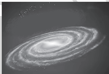
A C-19 jelű csillagáramlat fantáziarajza a Galaxis körüli keringésének egy pillanatában (Gemini Observatory/NOIRLab/NSF/AURA/J. da Silva/Spaceengine ; M. Zamani (NSF's NOIRLab))
