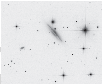
Sebestyén Attila fotója az NGC 4217 és NGC 4226 (tőle balra) látszólagos párosáról (15 T, ASI174MM, 60x120 s)
