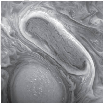
Két jellegzetes, kölcsönható örvény a Jupiter légkörében a 38. közelítés alkalmával, 2021. november 29-én (NASA/JPL-Caltech/SwRI/MSSS, Kevin M. Gill CC BY)
