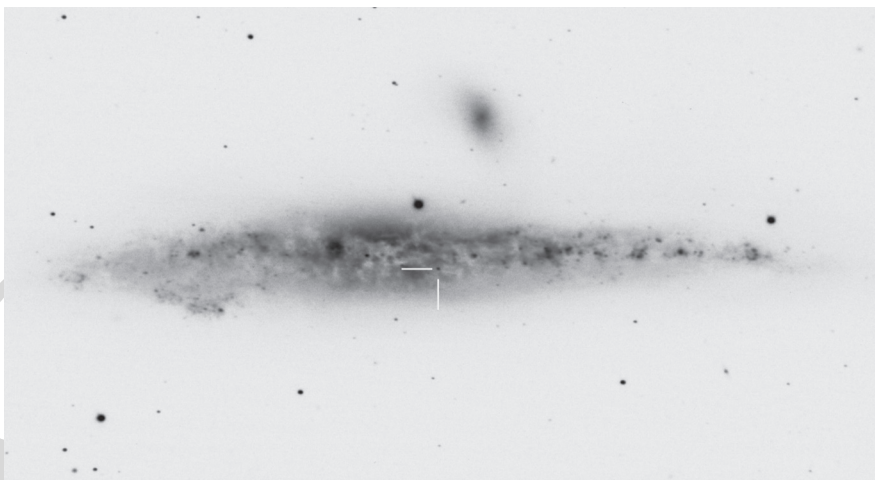
Az NGC 4631 és a benne robbant fényes vörös nóva, az AT 2021biy Molnár Iván felvételén (28 SC, Canon EOS 600D, 35x300 s, ISO 1600)
