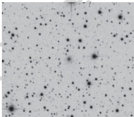
Sebestyén Attila 2020. november 7-i 10x60 s-os felvételén jól látszik a kompakt, planetáris kód kinézetű üstökös (150/750 T + ASI 174 MM)
