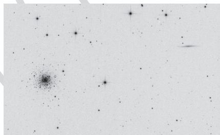
Sebestyén Attila felvétele az NGC 4147-ről (balra) és az UGC 7170-ről (jobbra). 150/750 Newton, ASI174MM kamera, 20x120 s
