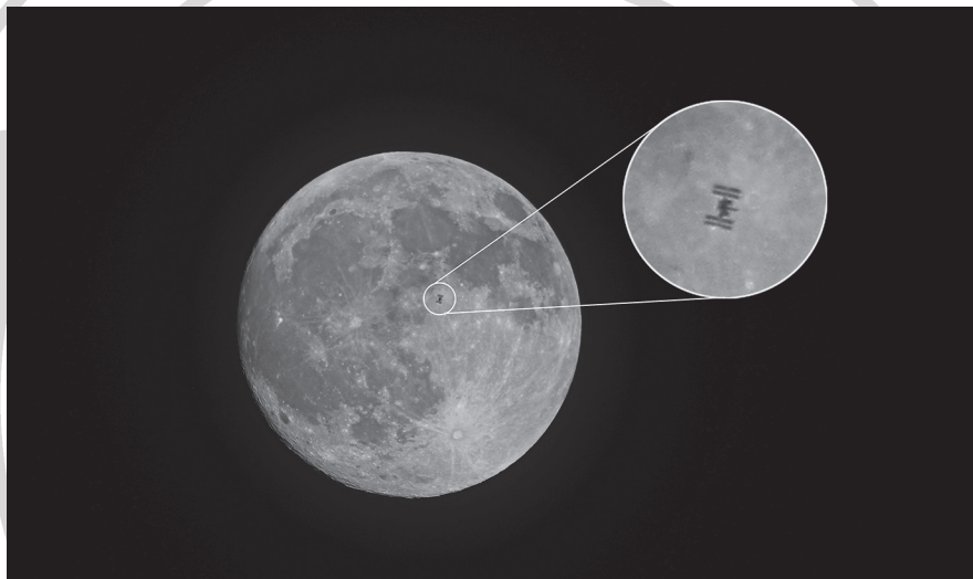
Óriásműhold a Hold előtt! A Nemzetközi Űrállomás 2020. január 10-én átvonult a Hold előtt Szalai Péter kisnyomú észlelőhelyéről nézve (bővebben l. a szövegben!)
