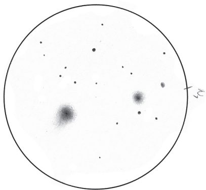
A rajzot Sánta Gábor az üstökös és az M87 együttállásakor készítette (150/750 L; 54x; látómező: 69 ívperc). Az üstökös a látómező keleti, míg a galaxis a nyugati széle felé látható
