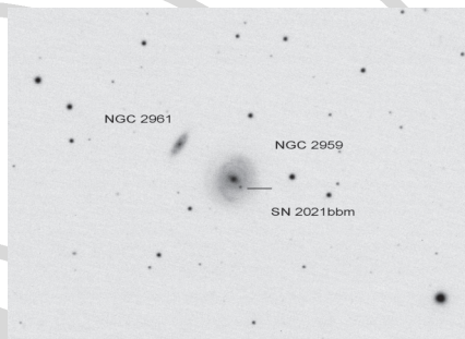
Az SN 2021bbm az NGC 2959-ben Molnár Iván fotóján (28 SC, Canon EOS 600D, 24 \times 180 s, ISO 1600)
