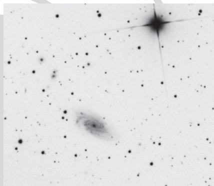
Az NGC 6070 a Kígyó csillagkép egyik legfényesebb spirálgalaxisa, Gerák Ferenc felvételén (20 T, ASI533, 52x180 s)
