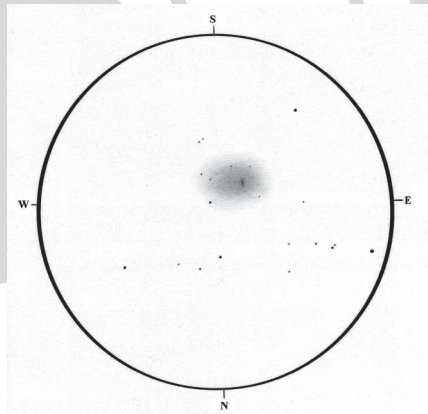
Kernya János Gábor rajza az NGC 6426-ről (35,5 T, 413x, 12')
