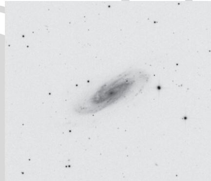
Sebestyén Attila fotója az NGC 3198-ről (15 T, ASI174MM, 70x120 s)
