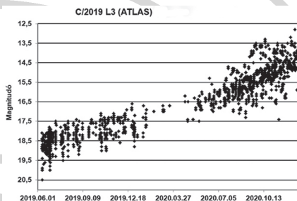
A C/2019 L3 (ATLAS)-üstökös fényességváltozása
