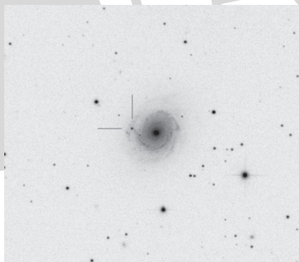
Sebestyén Attila felvétele az NGC 3147-ben robbant SN 2021hpr-ről (15 T, ASI174MM, 20x120 s)
