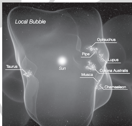
A Lokális Buborék fantáziarajza, a falban látható csillagkeletkezési régiókkal (Cfa / Leah Hustak (STScI))
