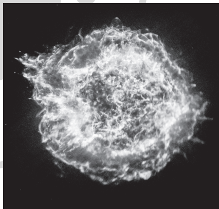
A Cassiopeia A szupernóva-maradvány (NASA/CXC/SAO)
