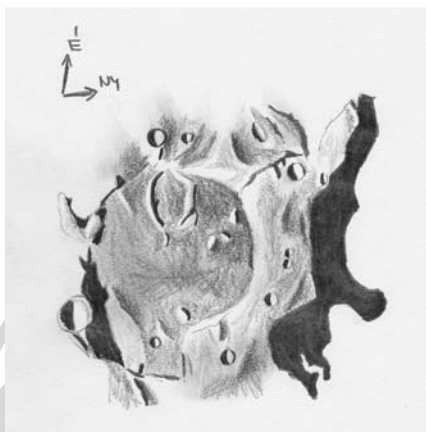
Ezt a rajzot Kárpáti Ádám készítette a Gauricus-kráterről 2022. február 11-én a 180/2700-as Makszutow-Cassegrain-teleszkópjával, 216x-os nagyítással, zenittükört használva
