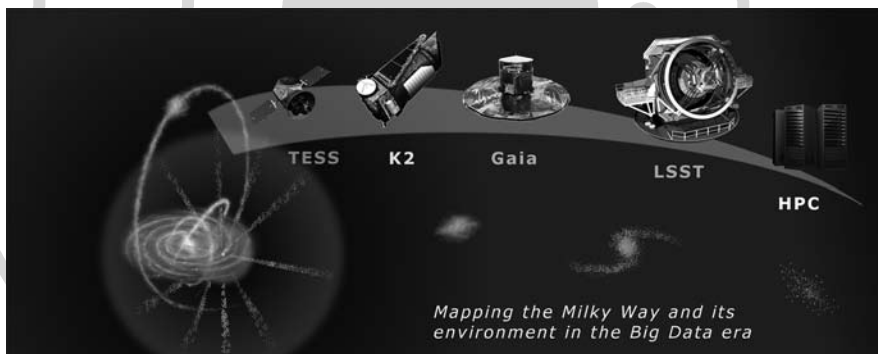
A szerző Lendület-pályázatának grafikus összefoglalása: űrfotometrián és nagy égboltfelméréseken keresztül a Tejútrendszer szerkezetének jobb megértése, valamint Big Data algoritmusok fejlesztése az LSST égboltfelméréssel kapcsolatban (Molnár László munkája)
