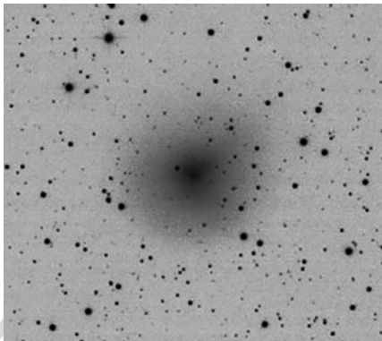
Jól kivehető a különböző időpontokban ledobott táguló anyagfelhők miatt létrejött réteges szerkezet üstökös kómájában. Sebestyén Attila felvétele 2021. november 9-én készült (203/1624 RC + ASI 174MM; gain 300; 60x120 s)
