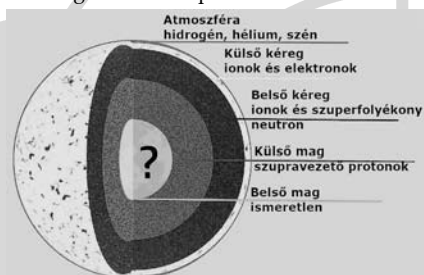
Egy „szokványos” neutroncsillag belső szerkezete (NASA's Goddard Space Flight Center/Conceptual Image Lab)
