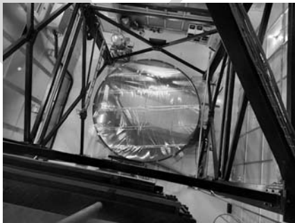
Az indiai ILMT védőfóliával borított higanytükrre (India Ministry of Science & Technology)
