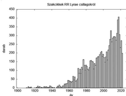
RR Lyrae csillagokkal foglalkozó szakcikkek száma évente az elmúlt 110 évben (NASA ADS)
