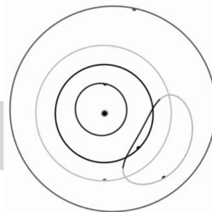
Az 2020 XL5 kisbolygó bonyolult mozgása. Az ábra a bolygók és a kisbolygó Földhöz rögzített koordinátarendszerben való mozgását mutatja. A XL5 kisbolygó a D alakú pályán mozog, pályája jelentős része a Vénusz pályáján belül húzódik, miközben maga a kisbolygópálya kis mértékben oszcillálva vándorol (Tony Dunn, Sky and Telescope, 2021. február 4.)
