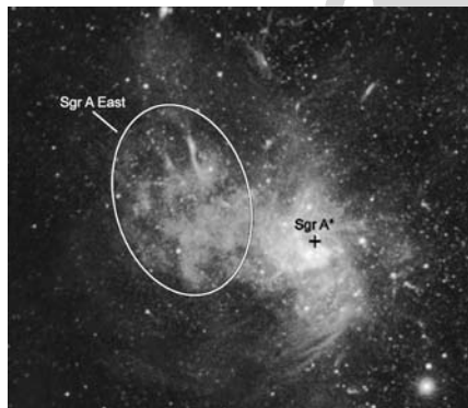
A feltehetően Iax típusú szupernóva-robbanásból származó Sgr A East nevű képződmény (NASA/CXC/Nanjing Univ./P. Zhou et al.; NSF/NRAO/VLA)
