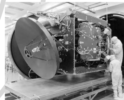
Az Al Amal összeszerelés közben (MBRSC / LASP)
