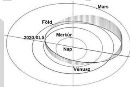
A 2020 XL5 kisbolygó pályája (NASA JPL SSD)
