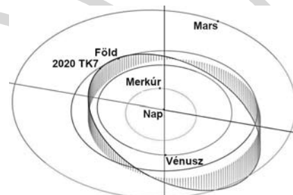
A 2010 TK7 pályája a Nap körül (NASA JPL SSD)
