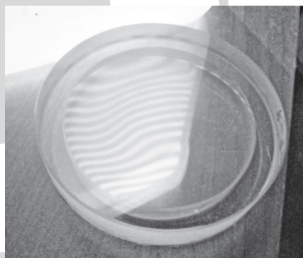
A segédтүкör ellenőrzésének egyik módja homorú gömb felületen való interferenciateszt. A képen az interferenciavonalak láthatók zöld fényben. Kellő tapasztalattal nagyon pontosan becsülhető, vagy akár mérhető is a felület alakja
