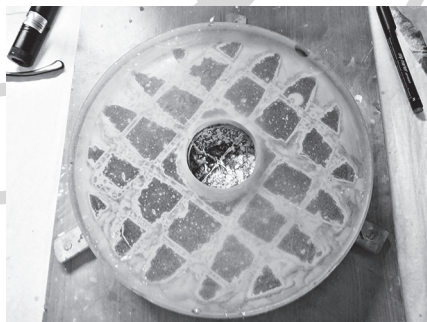
Nagy nyílásviszonyú tükrök esetén bevált módszer a fényezőtárcsa szegmenseinek a perem felé való „lekönnyítése”
