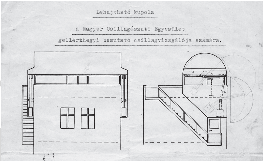
Lehajtható kupola az Urániára! Blahó Miklós okl. gépészmérnök, műegyetemi adjunktus elképzelése végül nem valósult meg
