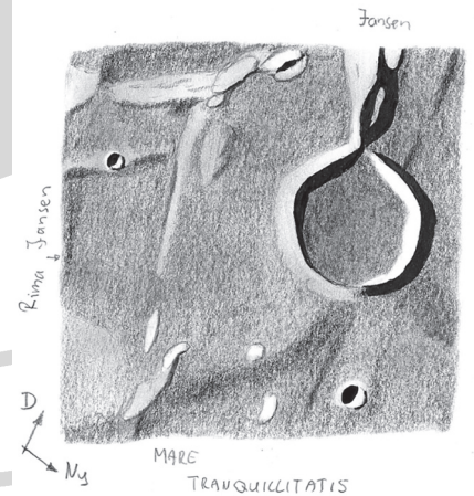
A Jansen és szűkebb környezete Görgei Zoltán 2000. február 10-én készült rajzán. A használt műszer egy 90/1000-es refraktor volt, 200x-os nagyítással
