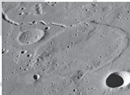
A lávával csordultig telt Jansen R-kráter és a Rima Jansen az Apollo-17 felvételén
