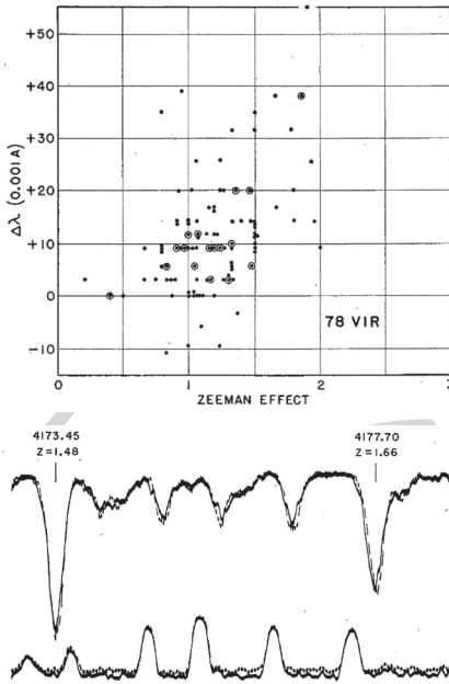
2. ábra. a) Egyedi vonalakra vizsgált eltolódások az elméletileg várt mértékű Zeeman-effektus függvényében a 78 Vir jelű csillag nagy diszperziójú (2,9 angström/mm) spektrumaiban. A bekarikázott pontok azokat az átlagértékeket jelölik, ahol a két különböző lemezen mért eltolódások 0,003 mm-en belül egyeznek
