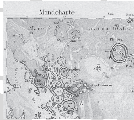
A Jansen-kráter Wilhelm Gotthelf Lohrmann nagyon szépen megrajzolt holdtérképén
