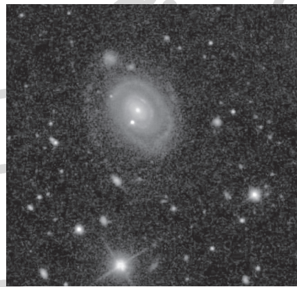
Az IC 75 az SDSS felvételén
