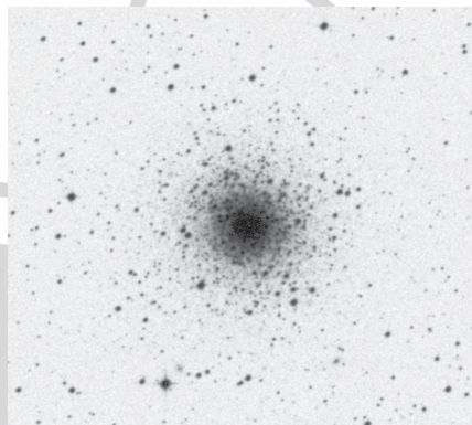
Az M75 a POSS2 vörös fényben felvett fotólemezen (10x10')
