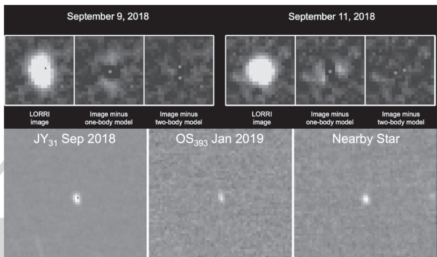
A Kuiper-övbeli két kettős kisbolygóról készült felvételek az objektumok elnyúltságát mutatják. Jobbra lent: egy csillag pontszerű képe referenciaként (NASA/JHAPL/SwRI)
