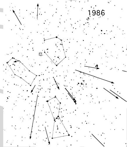
A Tepliczky István által 1986-ban látott néhány Aurigida meteor az akkoriban használatos meteorészlelő térképre rajzolva (Jenniskens utánközlése, 1997)
