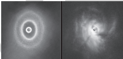
A GW Orionis rendszeréről készült felvételek. Balra: Az ALMA rádiótávcső-hálózat adatából nyert kép; jobbra: az ESO VLT távcsövén levő SPHERE műszer felvétele. A bal oldalon megfigyelhető a korong gyűrűs szerkezete, míg a SPHERE felvételén látható a belső gyűrű árnyéka (ALMA (ESO/NAOJ/NRAO), ESO/Exeter/Kraus et al.)
