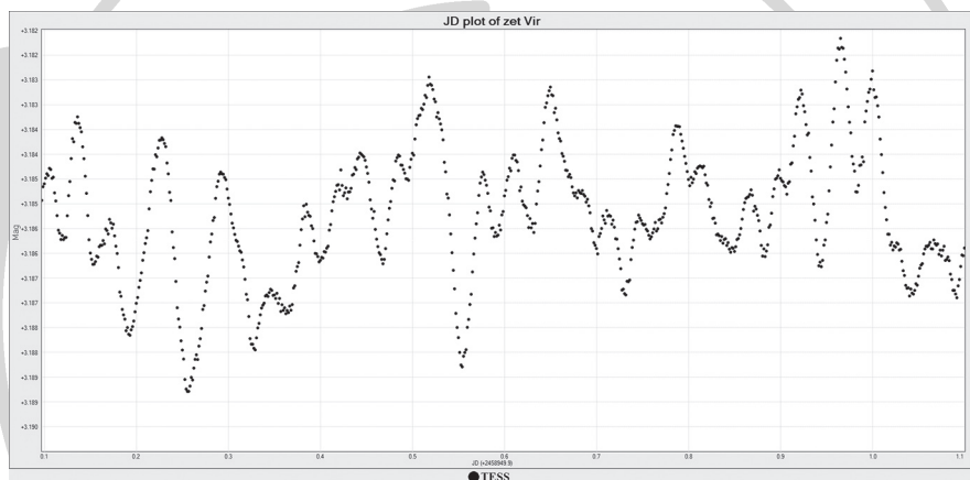
Egy nap a \zeta Vir fényességváltozásaiban, a TESS-űrtávcső adataiban. A bonyolult hullámzást többmódusú csillagpulzáció okozza (forrás: VSX)
