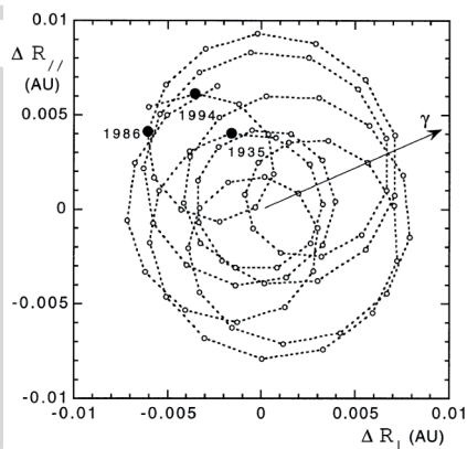
A Nap helyzete a Naprendszer tömegközéppontjához képest 1900 és 1995 között, CSE-ben kifejezve. Látható, hogy az első három ismert Aurigida-kitörés idején nagyjából ugyanolyan helyzetben volt a Nap, de az is észrevehető, hogy számos hasonló helyzetben nem volt kitörés (Jenniskens, 1997)
