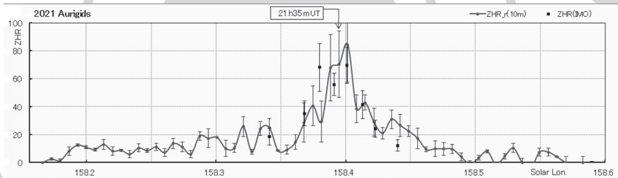
Az Aurigidák kitörésének rádiós grafikonja (Ogava Hiroshi és Sugimoto Hirofumi, IPRMO)
