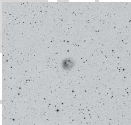
Az Abell 75 (NGC 7076) PL Cep a POSS2 kék fényben rögzített lemezén ( 10 \times 10' )
