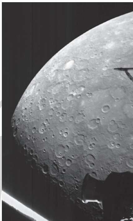
A BepiColombo október 2-án készített felvétele a Merkúr északi féltekéjéről (ESA, JAXA)
