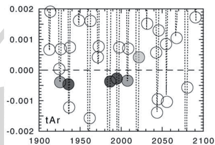
Az Aurigidák porsávjának számított távolsága a földpályától CSE-ben, 1900 és 2100 között azokban az években, amikor 300 ezer km-nél jobban megközelítettük azt. Sötétebb színnel a három ismert kitörést jelölték (1935, 1986, 1994), világossal pedig a cikk írásakor még előttünk álló 2007-es, illetve egy vélhetően elszalasztott 1926-ost. Utólag még halványabb színnel besatíroztuk az idei kitörést (Lyytinen & Jenniskens, 2003)
