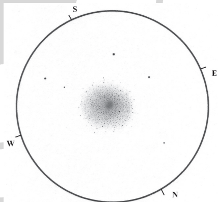
Az M75 Kernya János rajzán (35 T, 550x, 6')
