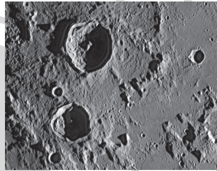
A Tempel-kráter Csabai István 2018. április 22-én készült nagyfelbontású holdmozaikjából. A Tempel a kép felső részén, központi csúcsos Agrippa-krátertől közvetlenül keletre (balra) található
