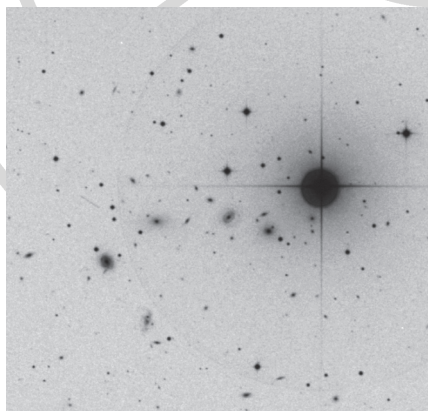
Az Abell 75 csoport a POSS2 kék fényben rögzített lemezén ( 10 \times 10' )
