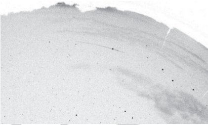
Az utolsó általunk látott, 23:53-as Aurigida a Bajai Obszervatórium teljeségbolt kamerájának 15 másodperces felvételén. Az északi horizont felett látszó meteor onnan nézve éppen eltalálta az \alpha UMa-t
