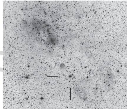
Az NGC 1946 (vonásokkal jelölve) a POSS2 vörös fényben felvett lemezén. Balra felfelé az NGC 1948 ködbe ágyazott csillaghalmazt látjuk, a látómező mérete kb. 20 \times 20'
