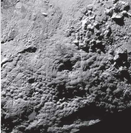
A kb. 155 km széles és 5 km magas Wright-hegység és a kép közepén látható gyűrű alakú struktúra (NASA/JHU-APL/SWRI)
