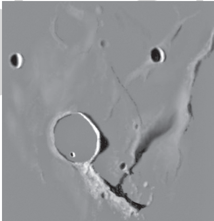
A Jansen-kráter és környezete Földvári István Zoltán 2021. szeptember 26-án, fogó fázisnál készült felvételén. Ez a szép digitális rajz egy 127/1500-as Makszutow-Cassegrain-távcsővel készült, 225x-ös nagyítás mellett
