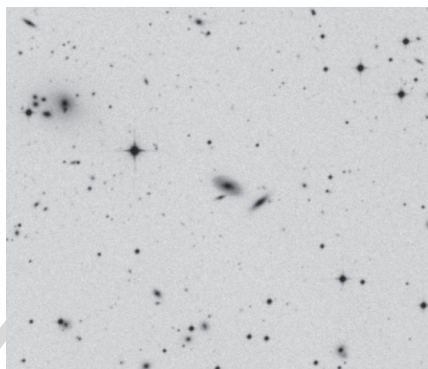
Az IC 1945-46, PGC 74537 csoport az Abell 3128 halmazban (Horologium csillagkép). POSS2 vörös fényben felvett lemeze, 10 \times 10'
