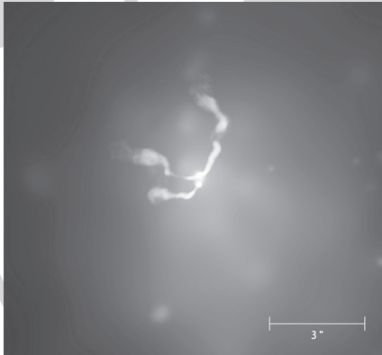
A 3C 75 kettős rádióforrás: jól látszanak az elkülönülő magok és a belőlük kiinduló, végük felé elgörbülő jetek is (kép: NRAO VLA)
