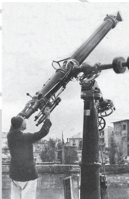
Az Uránia Bemutató Csillagvizsgáló főműszere, a 20 cm-es Heyde-refraktor 1947-ben. A szép műszer az épület tetején, egy 6x6 méteres teraszon kapott helyet. Egészen 1964-ig nem épült köré kupola, csak egy ideiglenesnek szánt bódé védte az időjárás viszontagságaitól
