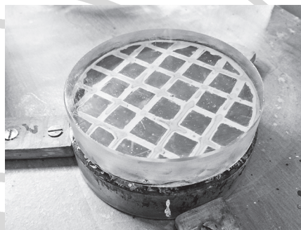
A segédтүкör ellendarabja a polírozótárcsán. Feltétlenül tökéletes gömbnek kell lennie, azonban teljes kipolírozása nem szükséges, mert csak referenciaként szolgál
