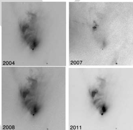
A McNeil-köd változásai 2004 és 2011 között (a Hawaii Egyetem 2,2 m-es távcsövével és a 8 m-es Gemini-North távcsövel Mauna Keaán készített felvételek, Colin Aspin nyomán)
