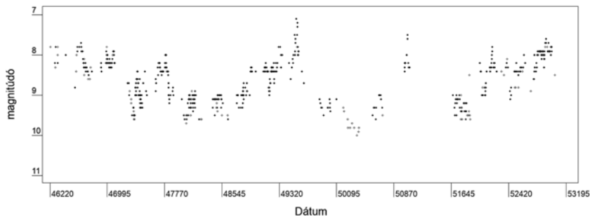
A CH Cygni szimbiotikus változócsillag fénygörbéje Sajcz András (Stz) észlelései alapján, 1985–2005 között. A csaknem 600 fényességbecslés nagyon jól kirajzolja a CH Cyg fényváltozásait (vcscs.mcse.hu)
