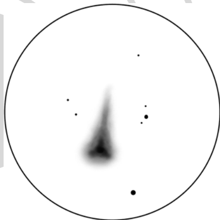
A C/1996 Q1 (Tabur) üstökös 1996. október 19-én 6,6 magnitúdós fényességnél (27 T, 60x)
