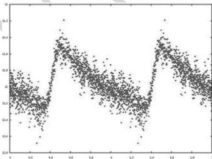
A BH Aurigae RR Lyr típusú változócsillag fénygörbéje a Légyszem mérései alapján
