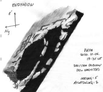
Az árnyékos aljzatú Endymion-kráter Fröhlich Viktória 2020. október 4-én készült rajzán. Az észleléshez használt műszer egy 200/1200-as Dobson volt, 120x-os nagyítással
