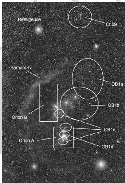
Az Orion csillagképről készült nagylátómezejű kép részlete, amelyen bejelöltük a szövegben említett régiókat. Zseli József felvétele alapján (Nikkor 85 mm-es objektív, Canon 6D fényképezőgép, 20x133 s, ISO 1000)
