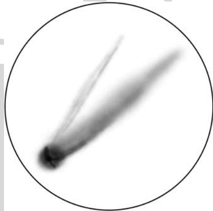
A C/1988 A1 (Liller)-üstökös 1988. április 15-én, 5,7 magnitúdós összfényességnél (15 T, 56x)
