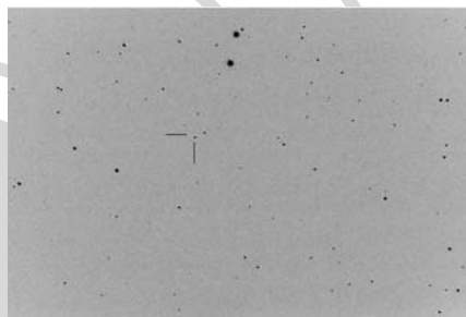
A PG1634+704 jelű kvazár felvétele a TAL200K-val 2018. október 31-én
