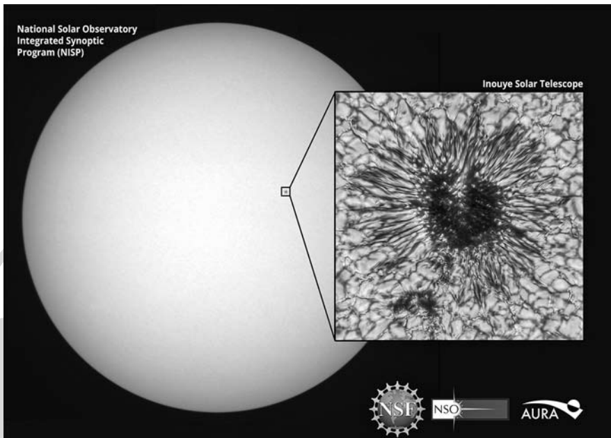
A David K. Inoye naptávcső rendkívüli részletességű felvétele a 2020. január 28-i napfotról (NSO/AURA/NSF)
