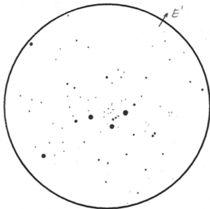
A Cr 69 Sánta Gábor rajzán (10x50 B, 5 fok)
