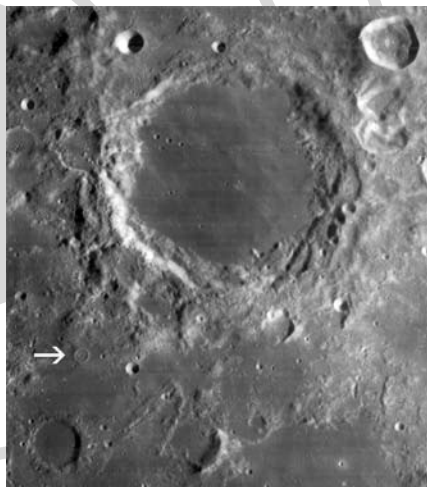
Ezt a felvételt is a Lunar Orbiter IV készítette. A kb. 7 kilométeres névtelen koncentrikus gyűrűs kráter a kép bal alsó részén látható
