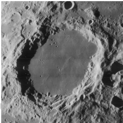
Az Endymion-kráter a Lunar Orbiter IV felvételén (fotó: NASA)
