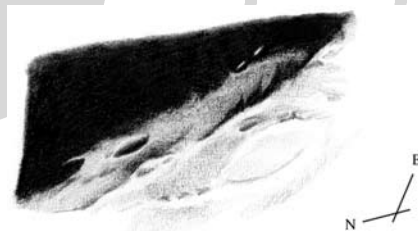
Ugyancsak 2012. december 29-én Földvári István Zoltán inkább az Endymiontól keletre húzódó hegyekre koncentrált. Az észleléshez használt műszer egy 80/910-es refraktor volt, 150x-es nagyítással
