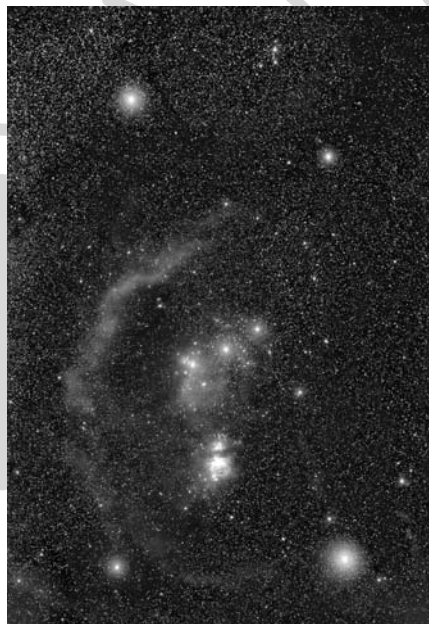
Zseli József nagy látómezejű felvétele az Orion csillagképről. Kiválóan azonosítható a Barnard-ív, amely az Orion–Eridanus szuperbuborék legfényesebb tartománya (Nikkor 85 mm-es objektív, Canon 6D fényképezőgép, 20x133 s, ISO 1000)
