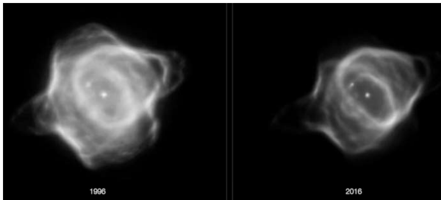
A Hubble-űrtávcső felvételei kiválóan mutatják a Hen 3-1357 jelű planetáris köd gyors halványodását mindössze két évtized alatt (NASA/ESA/B. Balick (University of Washington)/M. Guerrero (Instituto de Astrofísica de Andalucía)/G. Ramos-Larios (Universidad de Guadalajara))
