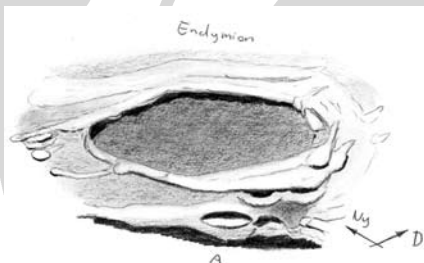
A rovatvezető 2020. december 1-én rajzolta le az Endymiont (90/1000-es refraktor, 250x-es nagyítás, zenittűkör)
