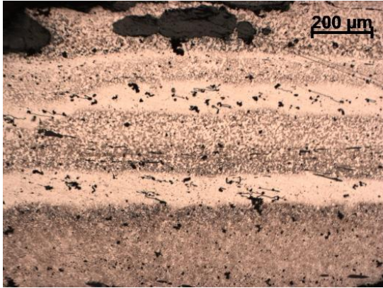
1. ábra: A Fülöp Gyula kard (Szent István Király Múzeum, Székesfehérvár/ltsz. n.a.) pengéjéből kimetszett minta a penge belső, mag részére eső területéről készült optikai mikroszkópos felvétel (készítette: Dr. Barkóczy Péter)
