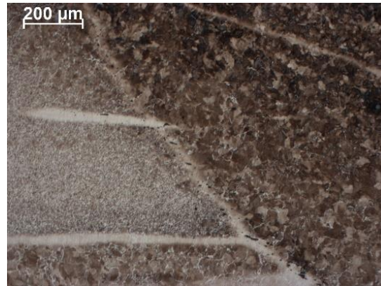
2. ábra: A kiskundorozsmai szablamarkolatú kard (Kiskundorozsma, Vöröshomok-dűlő, Móra Ferenc Múzeum, Szeged) mintájának éltoldásáról készült optikai mikroszkópos felvétel (készítette: Dr. Barkóczy Péter).
