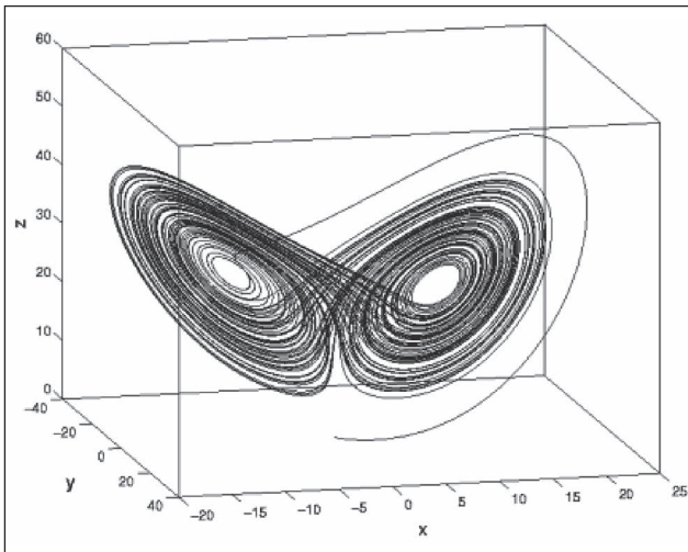
7. ábra. A Lorenz-attraktor (A szerző szerkesztése)
