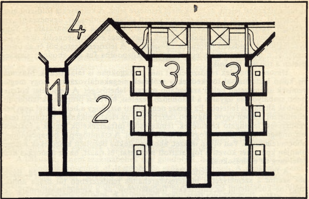
A szuperbiztonságú intézetek amerikai modellje. 1. Az őrség folyosója; 2. zárkacsarnok; 3. zárkák; 4. tetőablak.
