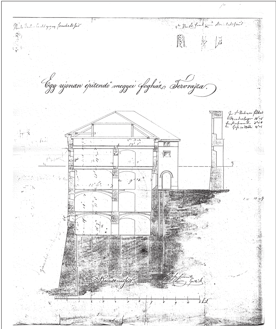
A Veszprémben építendő megyei fogház tervanyagának keresztmetszeti tervlapja Szász Ferenc tervéből, 1846. Országos Levéltár (MOL-D-112)
