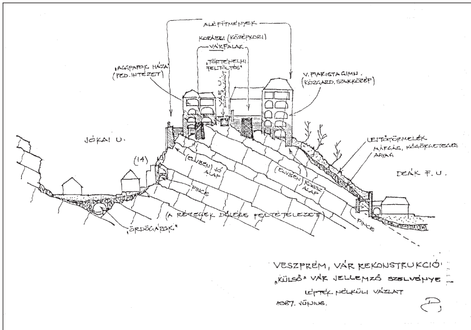
A veszprémi Külső-Vár vázlatos keresztmetszévény. Balassa László rajza.
