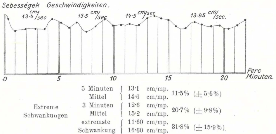
Fig. 21. Schwankungen der Wassergeschwindigkeit während eines Zeitraumes von 22 Minuten. 26. September Nördlicher Arm.
