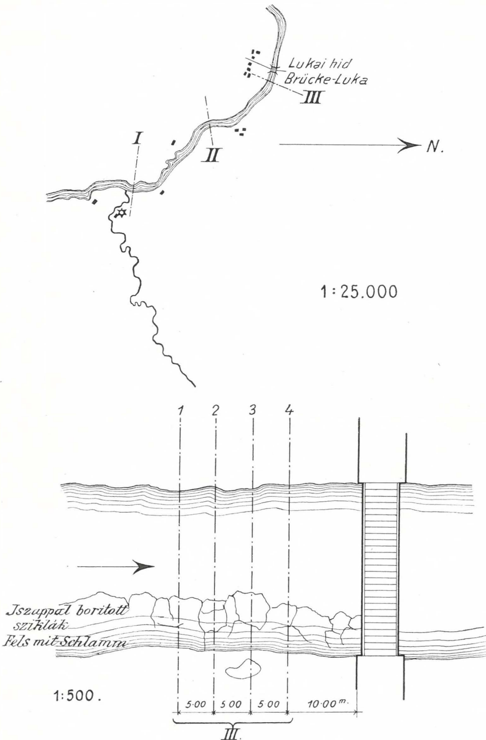
Fig. 10. Situation der am 30. Juli geyeilten Querprofile (gemeinsame Gačka); Querprofile III oberhalb Luka-Brücke.
