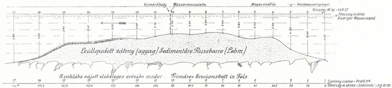
Fig. 9. Längenprofil nach der Tiefenlinie in Figur 8. Längen 1 : 500. Tiefen 1 : 100.
