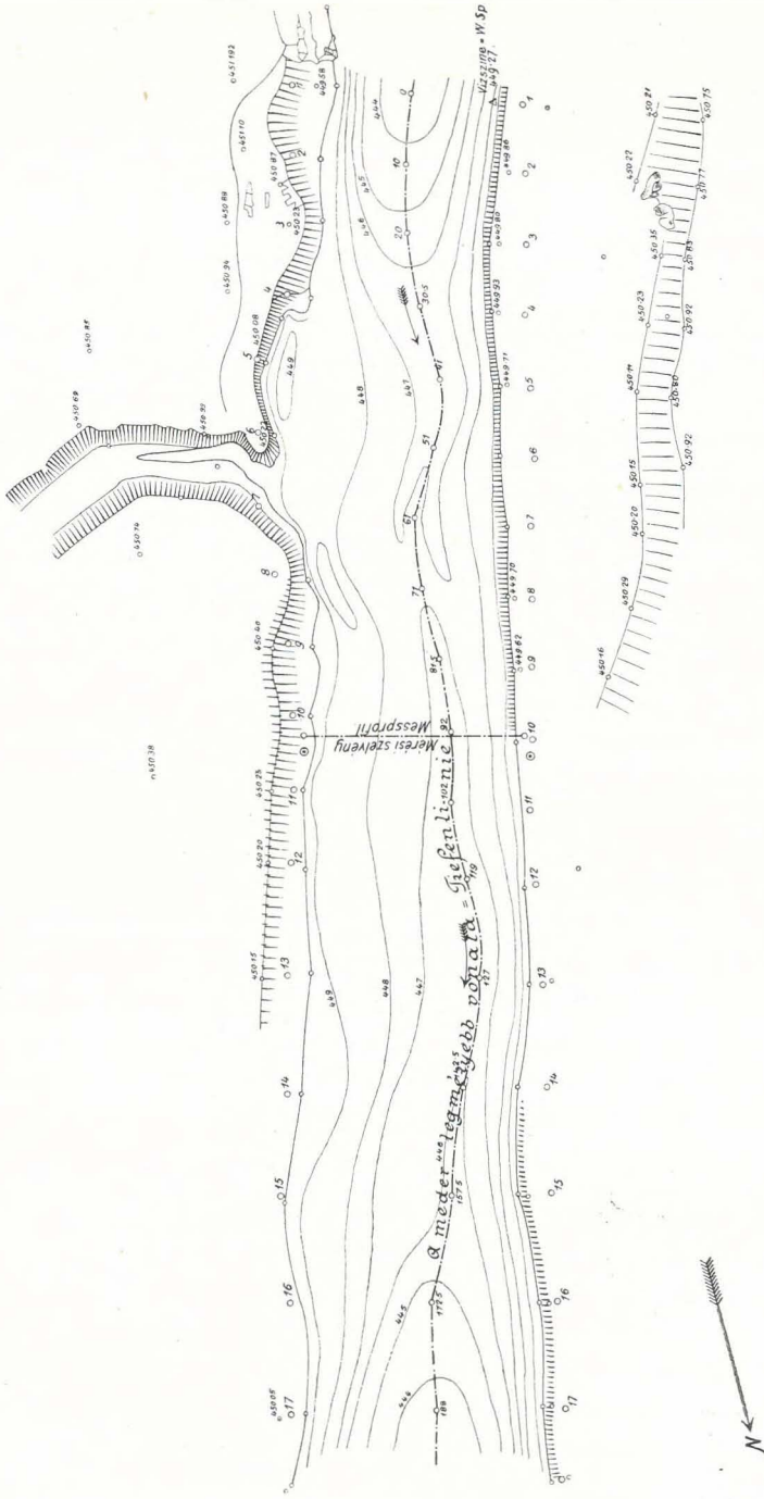
Fig. 8. Situation der Wassermeßstelle bei Prozor. Aufgenommen bei einem Pegelstand 47.50 (Pegel Luka).
