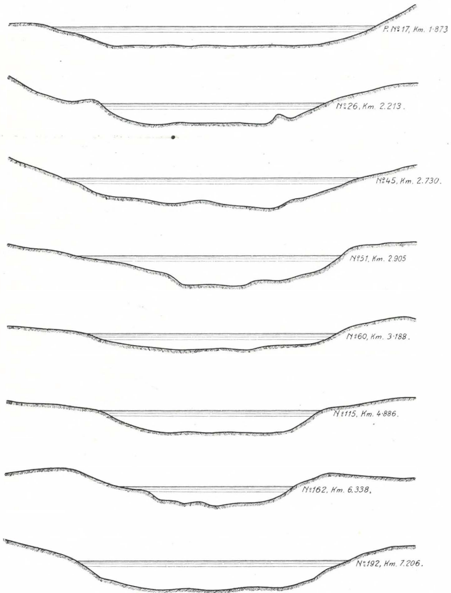
Fig. 15. Charakteristische Querprofile des nördlichen Gačkaarmes. Bezogen auf Mittelwasser I. ( 10 \text{ m}^3/\text{sec sec} gemeinsamer Arm). Maßstab 1 : 200.
