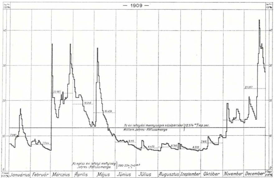
Fig. 24. Wasserführung des Gačka-Flußes.
