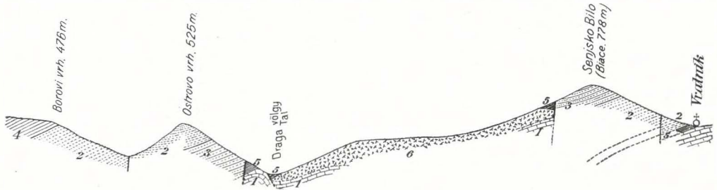
Fig. 27 Geologisches Profil A—A: vom Vratnikpaß bis zum Borovivrh. Zeichenerklärung siehe bei Figur 26.
