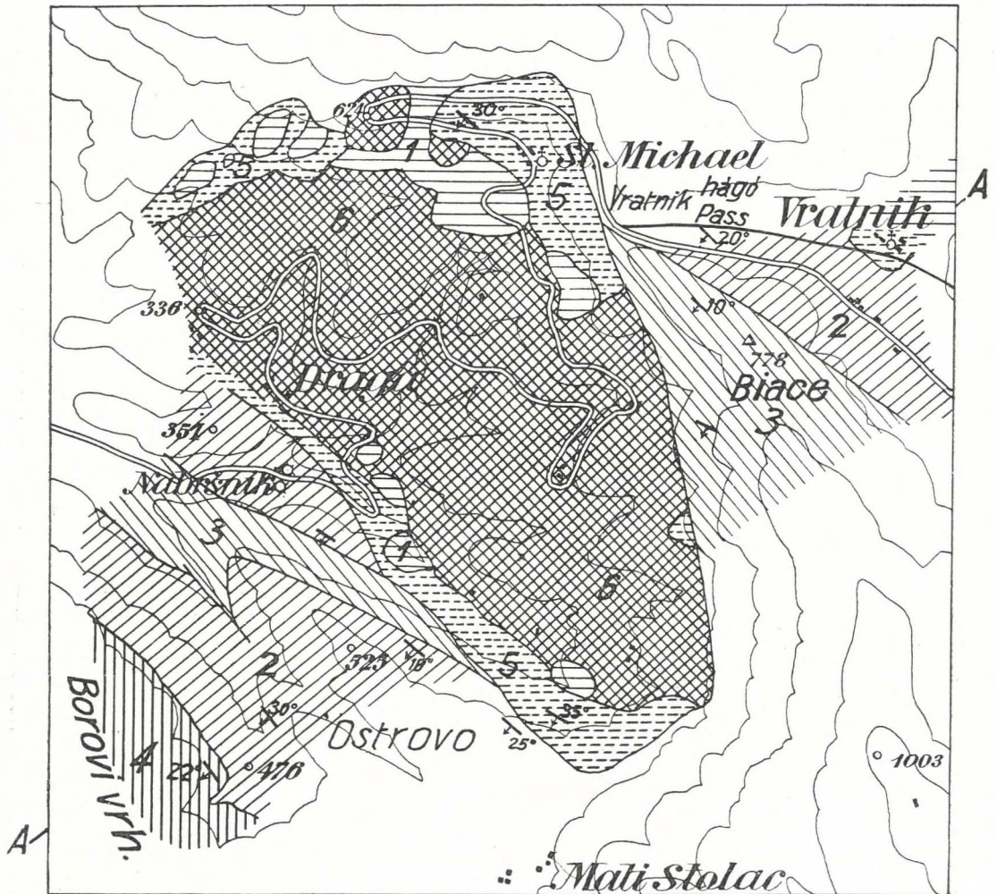
Fig. 26. Geologische Karte des Dragatales.
