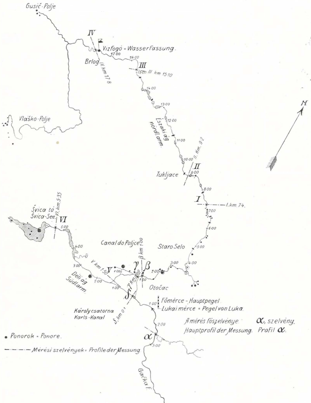
Fig. 6. Übersicht über die im Gačka-Gebiet auftretenden Schluckschlünde.
