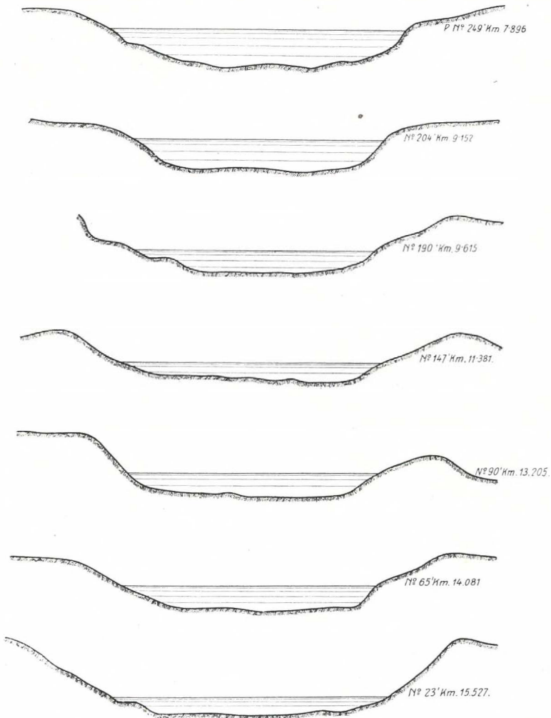
Fig. 15. Charakteristische Querprofile des nördlichen Gačkaarmes. Bezogen auf Mittelwasser II. ( 10 \text{ m}^3/\text{sec} gemeinsamer Arm). Maßstab 1 : 200.
