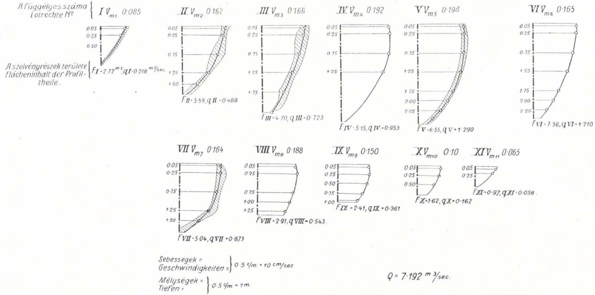
Fig. 20. Wassermessung No 16 Prozor, Meßprofil \alpha , September 1909, Pegel Luka : 50.5.
