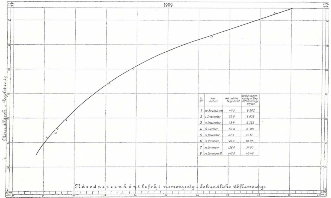
Fig. 23. Konsumtionskurve für den Gačkafluß bezogen auf Pegel Luka.
