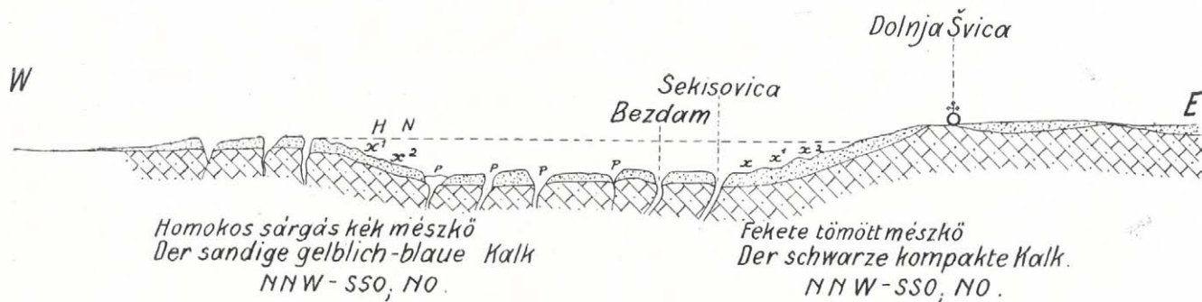
Fig. 2. Profil. durch den periodischen Švica-See nach Prof. Cvijić.
