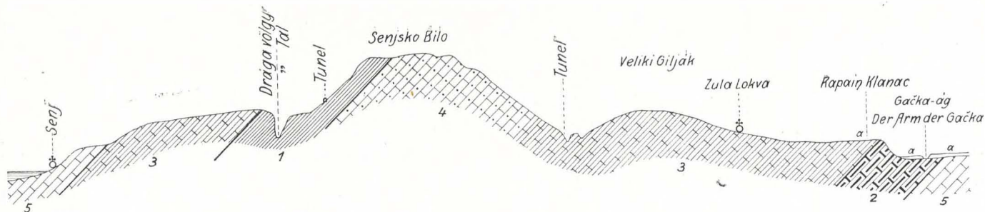
Fig. 1. Geologisches Profil von Brlog bis Senj nach Prof. Cvijić.
