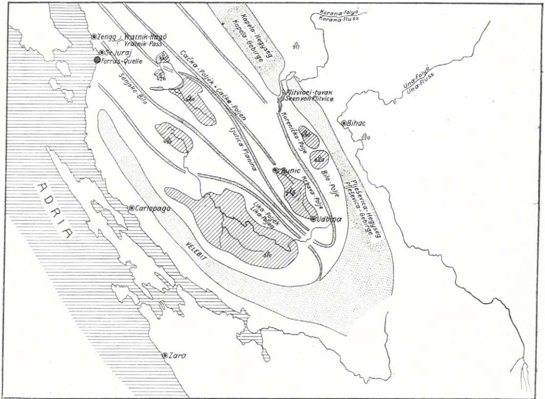
Fig. 5. Orographische Übersicht über das innerkroatische Hochland.
