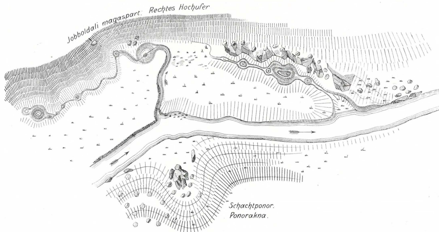
Fig. 17. Ponorlandschaft in km 2·5 des nördlichen Gačkaarmes.
