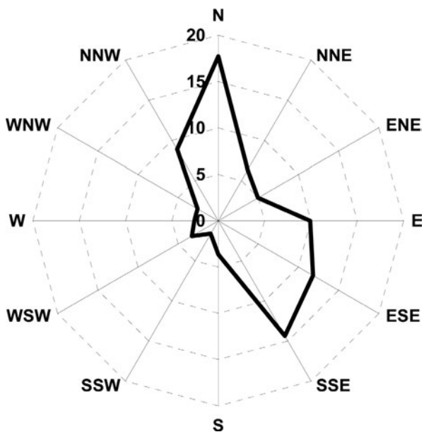
Szélirány-gyakoriság (%) 1995 - 96. tél Veszprém - Szentkirályszabadja repülőtér
