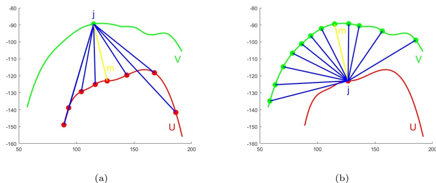
5. ábra. Az NND távolságmérték grafikus reprezentációja
