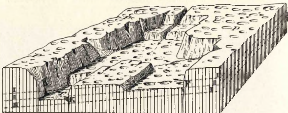
3. ábra. — Ideiglenesen vagy állandóan elárasztott polje. P = A magas planina. T = Állandó vagy időszakos tó. K = Katavotrák. F = Időszakos ferrás. I = Árvíz. II = Középvíz. III = Kisvíz.
