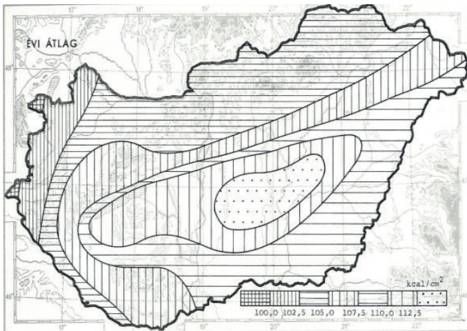
4. ábra. (fenn) A napsütés (óra) évi összegének területi eloszlása, 15 évi átlag (1958-72) (Major, 1985), (lenn) a globálsugárzás (kcal/cm 2 év) évi összegének területi eloszlása, 15 évi átlag (1958-72) (Major, 1985).
