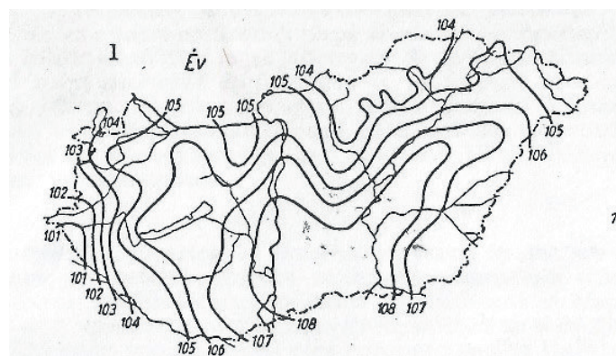
2. ábra. A besugárzás ( Kcal/cm^2\text{év} ) évi összegének területi eloszlása, 50 évi átlag (1901–50) (Dobosi és Takács, 1959).
