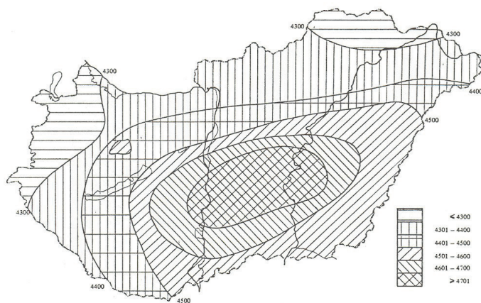
5. ábra. A globálsugárzás évi összegeinek területi eloszlása 1951-80 időszakra MJ/m 2 -ben (Dávid et al., 1990).
