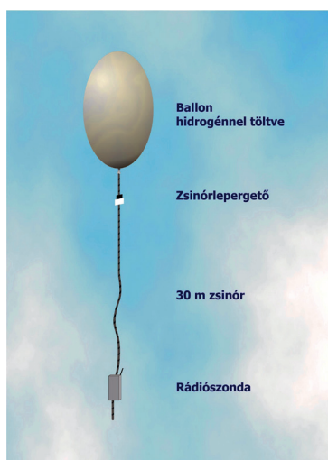
4. ábra. Hazánkban jelenleg használt rádiószonda szerelvény.
