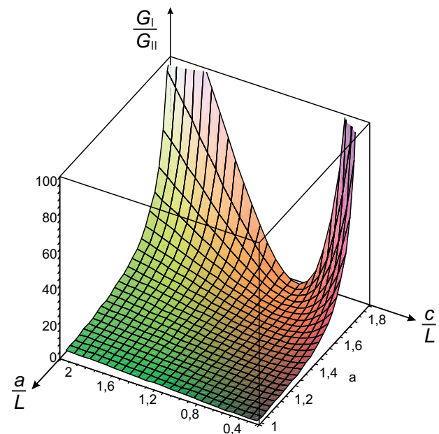
4. ábra. A módusok arányának változása az MMB próbatételnél az a/L és c/L viszonyok függvényében.
