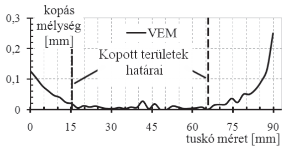
12. ábra. Végeszelemes számításokkal kapott, és mért értékek összehasonlítása 100 s esetén
