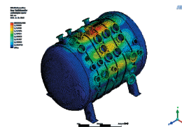
Végelem analízis
