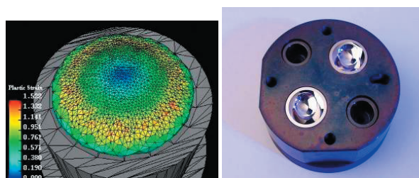
8. ábra. Szimuláció és az elkészült szerszám
