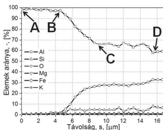
3. ábra Al99,5 mátrixú, SL150 típusú mikrogömbhéjakat tartalmazó szintaktikus fémhab vonalmenti EDS vizsgálatának eredménye
