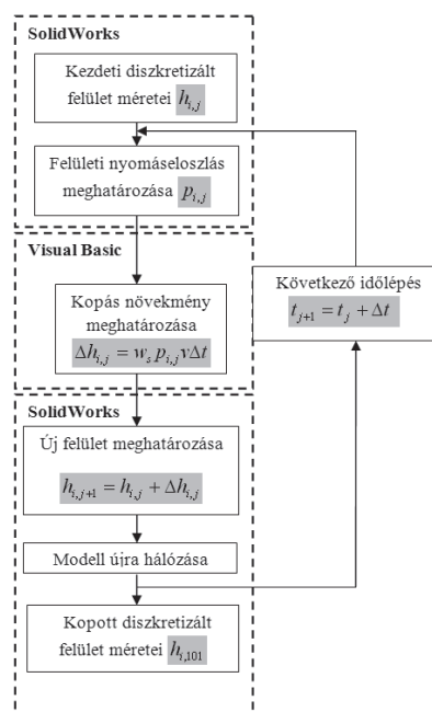
9. ábra. A kopászámítás elvi folyamatábrája
