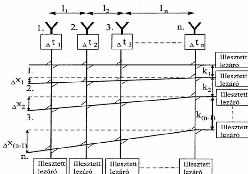
7. ábra. Mátrix típusú nyálábeltérítés
