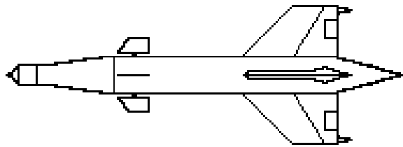
3. ábra. Fordított (kacsza) aerodinamikai elrendezés
