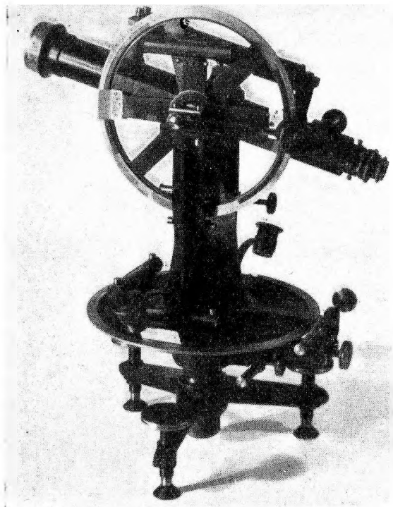
9. ábra. Régebbi típusú teodolit.
