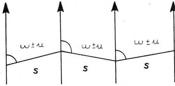
7. ábra. Függő kompaszsal történő poligonmérés.
