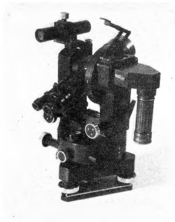
10. ábra. Zeiss 01 típusú teodolit.
