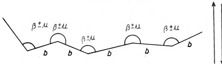
8. ábra. Teodolittal történő poligonmérés.
