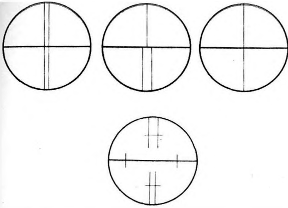
Fent balról jobbra: 12., 13. és 14. ábra, alul 15. ábra. Szálkereszt típusok.
