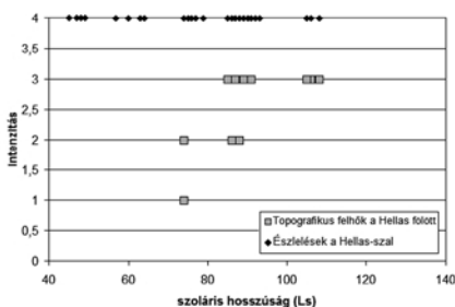
c Topografikus felhők előfordulása a Hellas medencéje fölött
