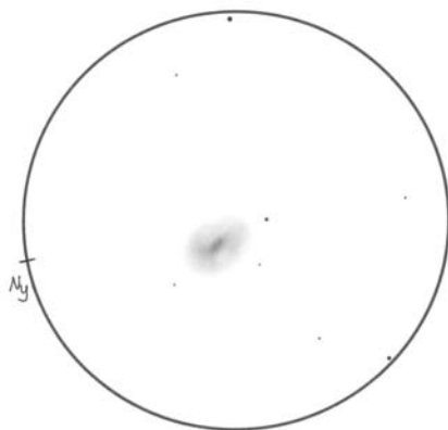
Az NGC 4214 Sánta Gábor rajza. 220/1200 T, 133x, 25'
