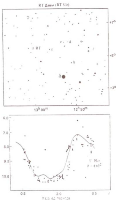
Az RT Vir szovjet észlelőtérképe és az U Her fénygörbéje odesszai fotografikus észlelések alapján
