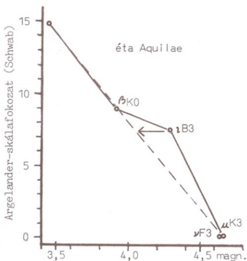
1. ábra. Az éta Aql összehasonlítóinak magnitúdó—skálafokozat összefüggése. A pontok mellett a csillagok jelölése és színképtípusa olvasható. Feltűnő, hogy a kék színű B3 típusú iota Aql kiugrik a sárga (F) és vörös (K) csillagok sorából.
