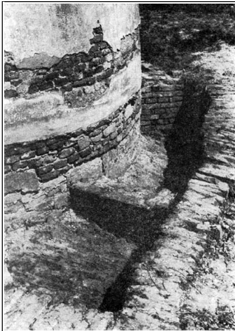
18. A vízvezető-rendszer a szentély falával
