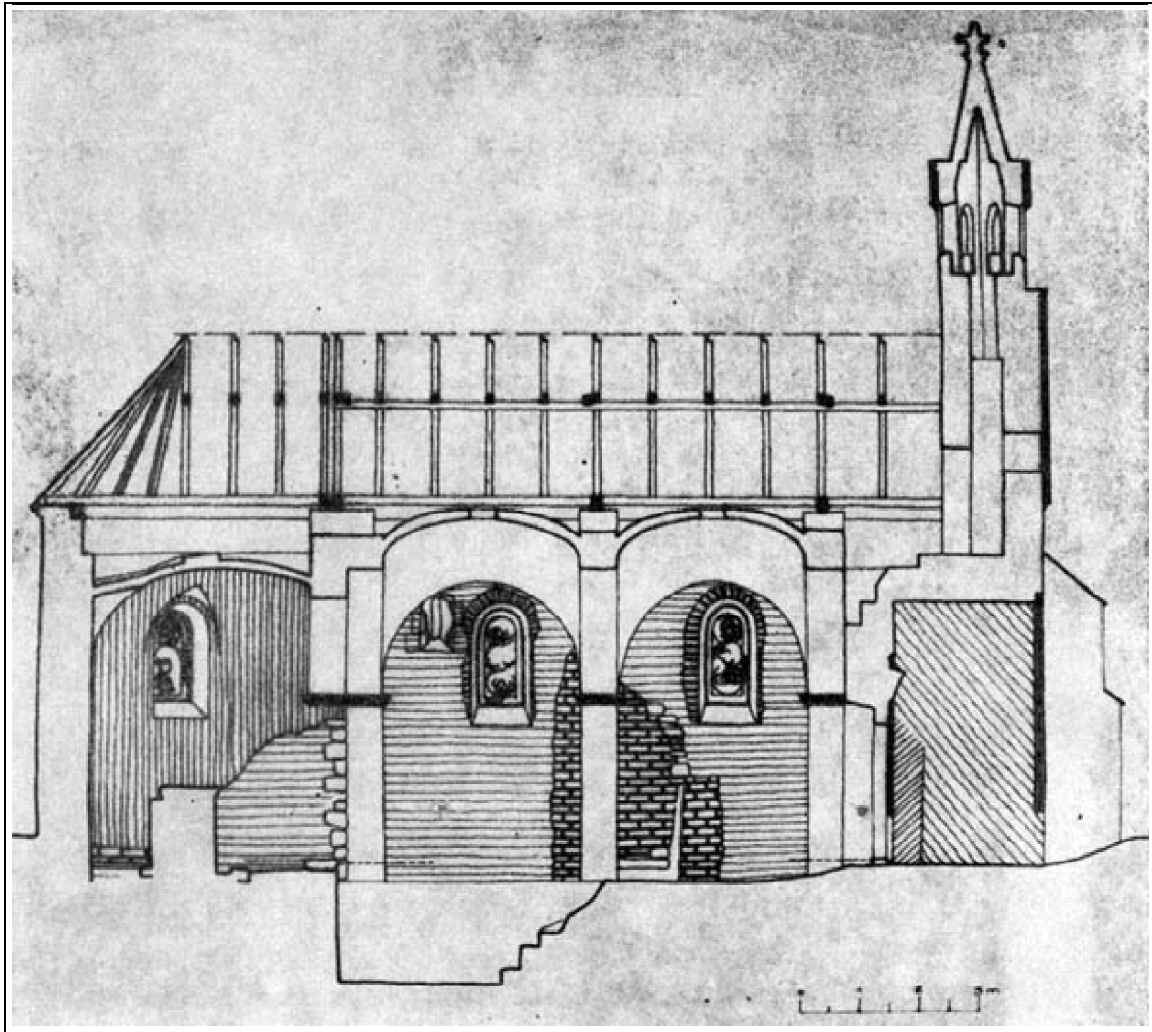
9. A templom keleti-nyugati metszete a kutatás eredményeivel
