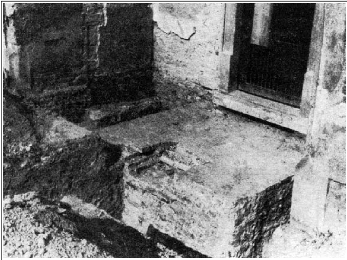
17. A tervezett nyugati torony alapozása
