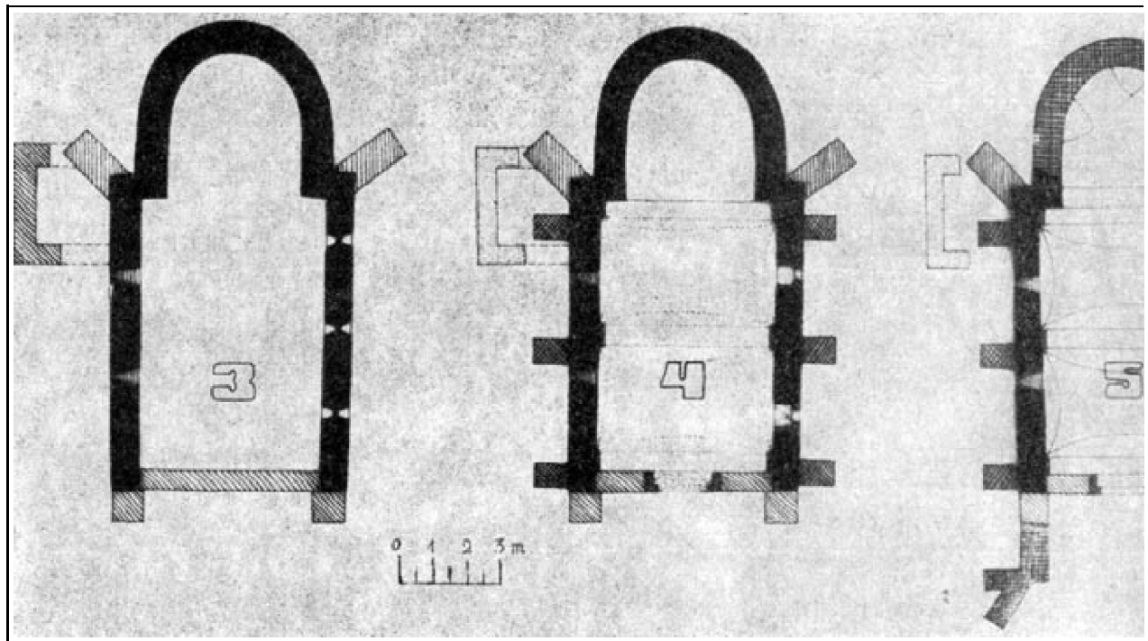
2935. A templom építési periódusai
