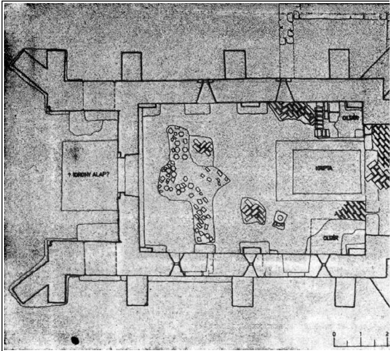
30312. A templom kutatási alaprajza
