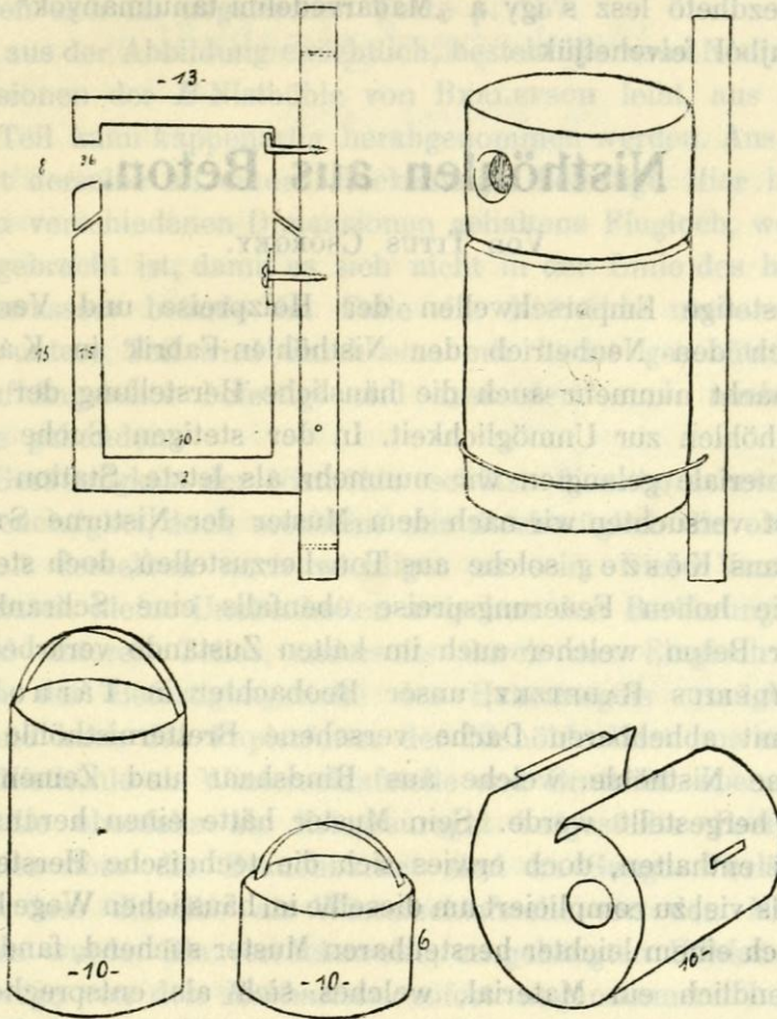
6. ábra. Cement-fészekodu és öntőminta.
