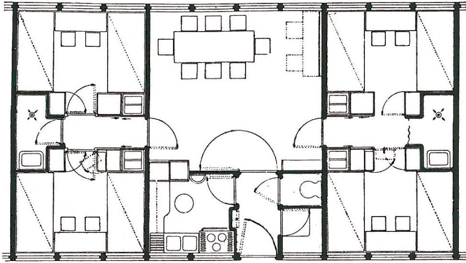
4. kép: Molnár Farkas terve: 70 m 2 -es lakás 8 ágygal. Tér és Forma , 1930, 1, 11
