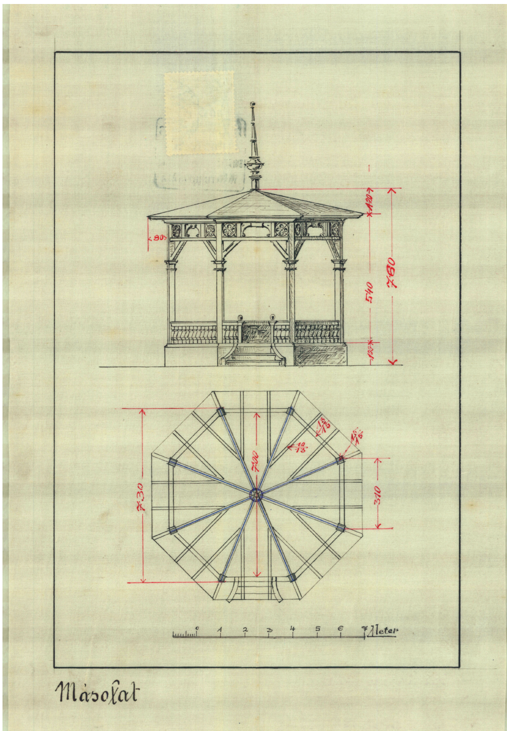
27. A nyolcszögletű vasszerkezetű pavilon alaprajza és nézete. Szerző nélkül, év nélkül. BFL XV.17.d.325 40/2
