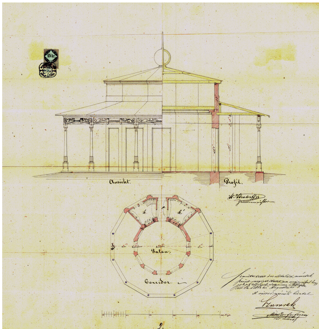
3. Alaprajz, metszet és nézet. Strohofer István, 1862. BFL XV.17.b.314 77/c a terv megegyezik a BFL XV.17.b.312 ÉB 3/1863 számú lappal
