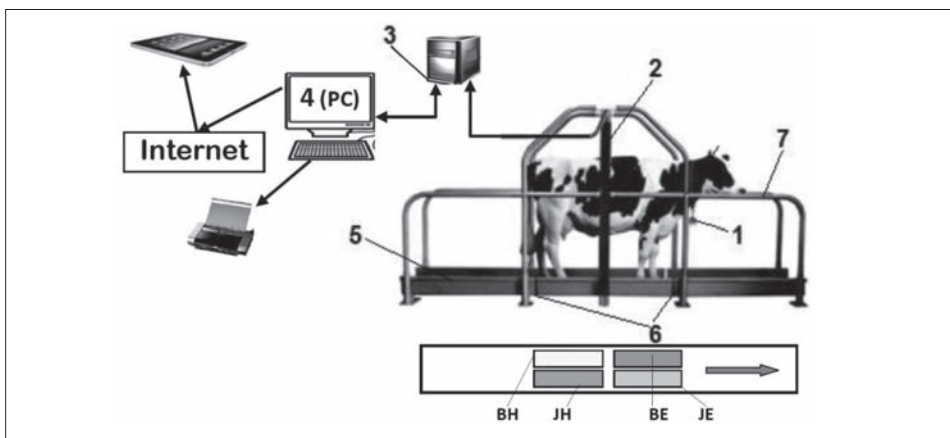
8. ábra STEP Metrix (Bou Matic) rendszer elvi felépítése ( http_1 , szerkesztette Tóth, 2013)
