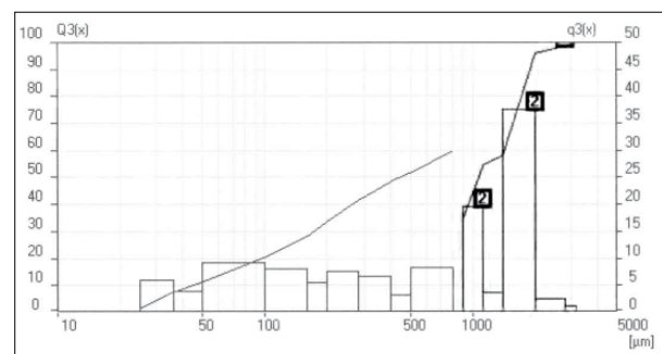
4. ábra A 4. rostfrakció minta vizsgálatának eloszlási grafikonja – Q3(x) súlyeloszlás (%); q3(x) sűrűség eloszlás (%)
