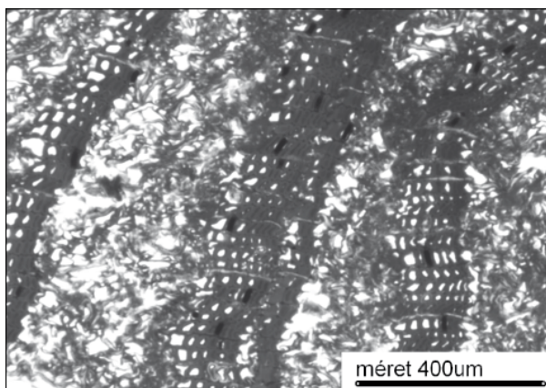
6. ábra Hossztracheidák szabályos elrendeződés (5-ös minta) Figure 6 Regular pattern of longitudinal tracheids (sample nr. 5)
