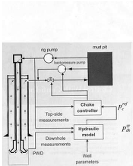
20. ábra: Számítógépes vezérlés elve
