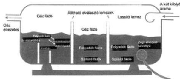
15. ábra: Négyfázisú szeparátor
