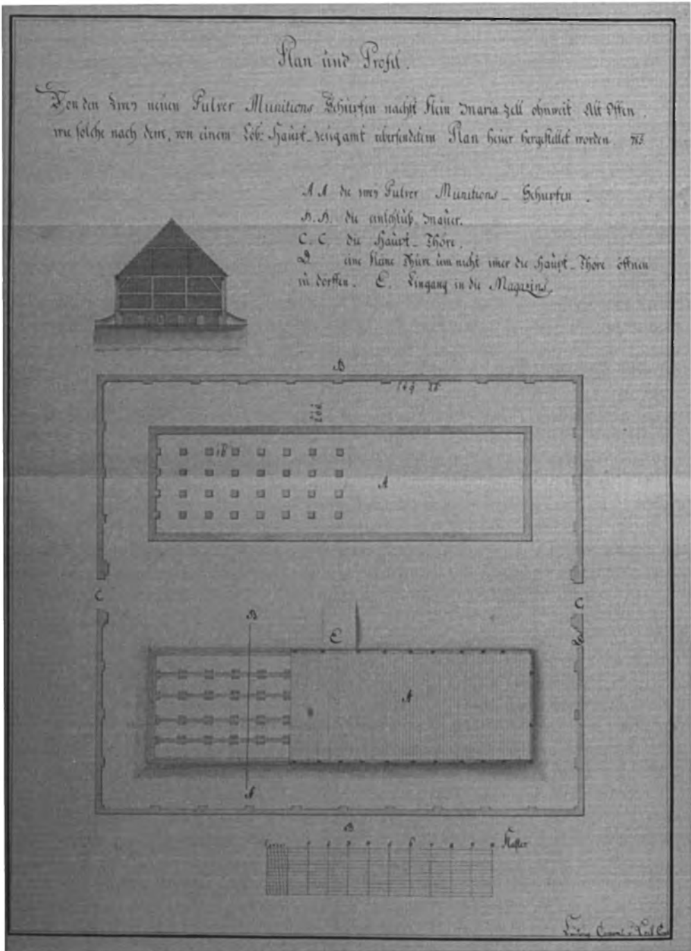
A kiscelli löporbarakk terve, 1786. Készítette: Ludwig tizedes (Österreichisches Staatsarchiv, Kriegsarchiv, Kartensammlung, GVII, 1806-D-67)
