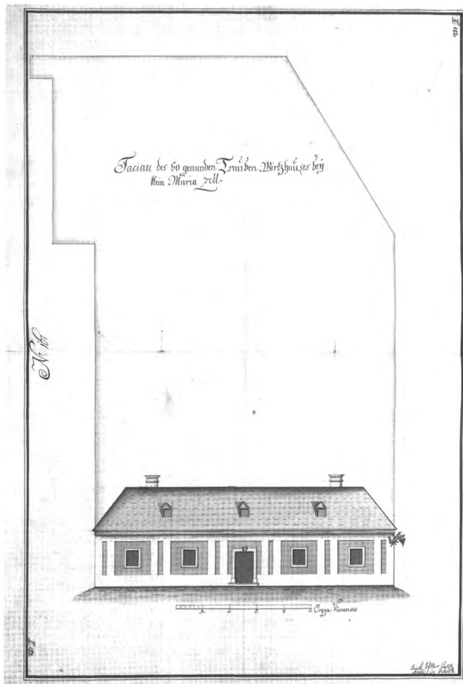
A kiscelli fogadó felmérési rajza, nyugati homlokzat és befoglaló alaprajz, 1774. Készítette: Jacob Gföller gödöllői kamarai építész (MOL, T1 szekció, No. 182/2)
