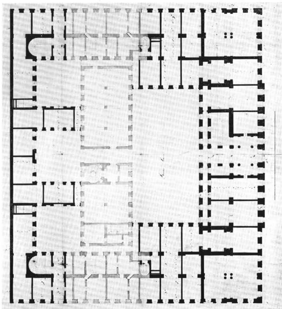
13. A lipótvárosi Valeró-gyár földszintjének alaprajza Hild Józseftől.
