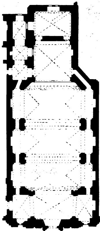
7. A karmelita-templom alaprajza.
