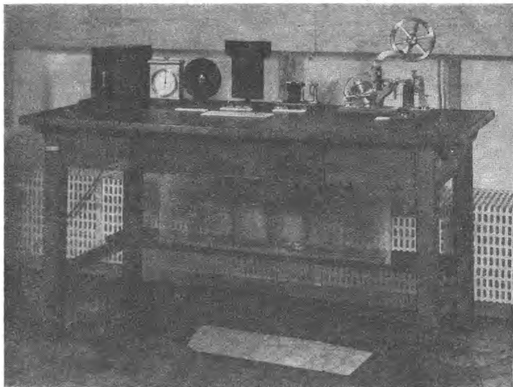
3. Középállomási táviróasztal, rugóműves dombfőgéppel, jelfogóval, dugaszos vonalváltóval és szalag tárcsával, 1900 körül. Telegraphentisch mit Fernschreibapparat und Relais, um 1900
