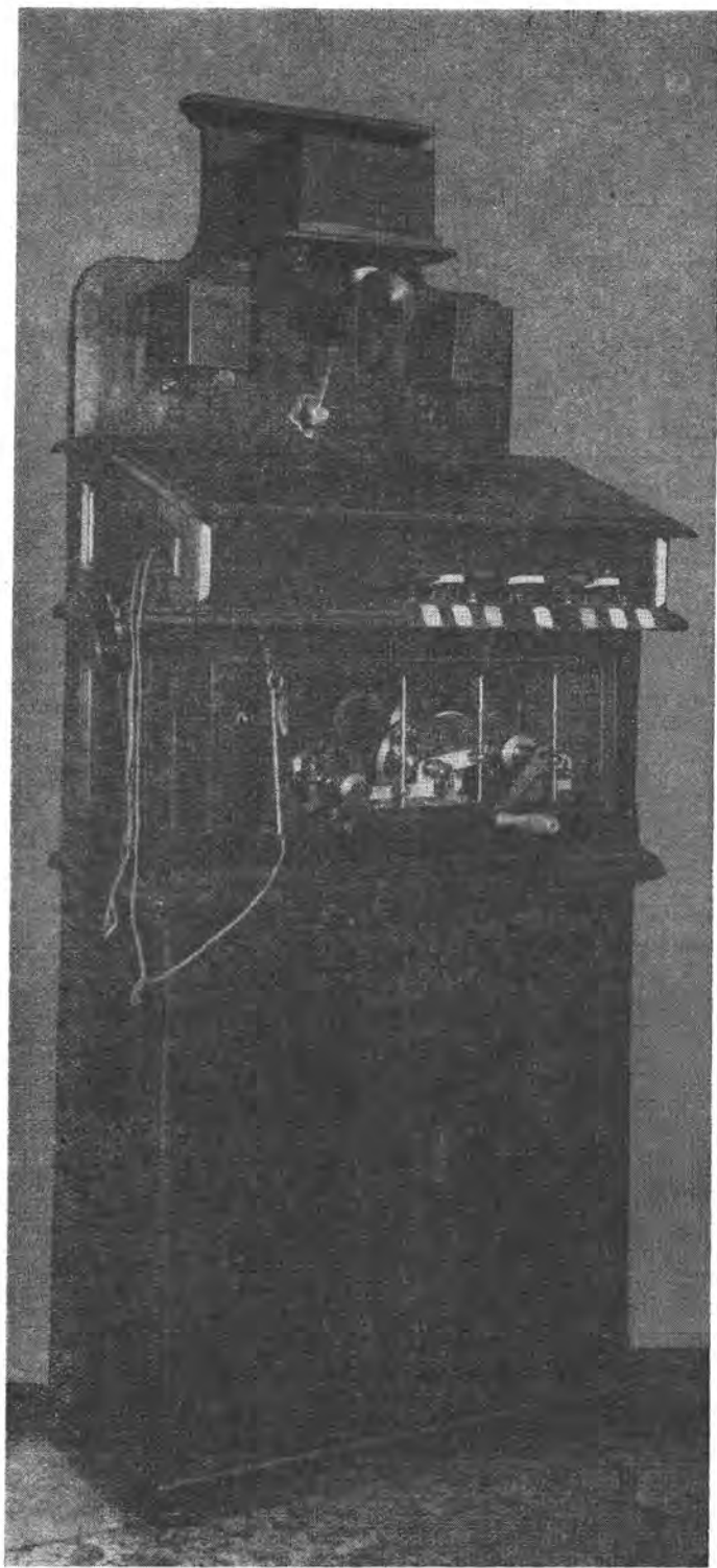
1. Telefonnal is felszerelt, indukált árammal működtetett állomási harangjeladó és jelzőállító berendezés, 1890. Glockensignalapparat mit Telephon für Eisenbahnen im 1890
