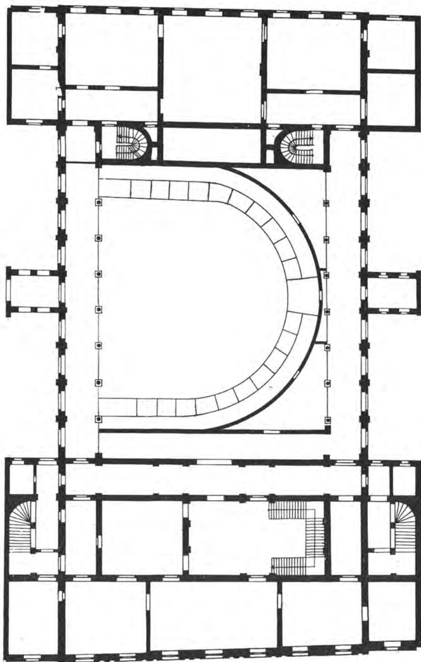
17. kép. A régi képviselőház I. emelete
