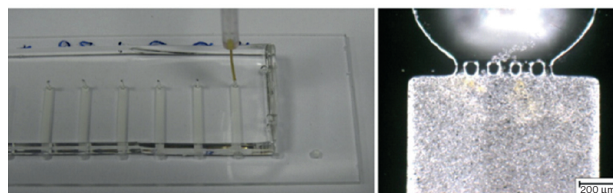
2. ábra. Mikrofluidikai chip egy lehetséges kapcsolása LIBS detektálással, kis térfogatú (nL–μL) folyadékminták előkezelésére, például fémionok kromatográfiás elválasztására. A mikrofluidikai chipből kifolyó folyadék a mikroszkóp tárgylemez-hordozójában kialakított kis gödörben gyűlik össze és szárítható be. Ezután a LIBS-mérés végrehajtható rajta. D = fénygyűjtés iránya, L = gerjesztő lézernyaláb iránya
