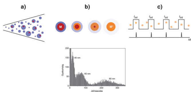
4. ábra. Az egyrészcseke ICP–MS módszer jelképzése. Felső sor, balról jobbra: a) nagyon híg vizes közegű nanodiszperzió-minta beporlasztása, cseppekre szétosztása, b) a plazmában való áthaladáskor a cseppek oldószertartalmának elpárolgása, a részecskék lebomlása és ionizációja, c) alkalmasan megválasztott integrációs idő mellett a detektor az egyes részecskéktől származó jelcsúcsokat külön regisztrálja. Alsó sor: a jelcsúcsok magassága a részecskékben található anyagmennyiséggel, vagyis a mérettel (térfogattal, tömeggel) arányos; hisztogramon gyakoriság szerint ábrázolva a jeleket, kirajzolódik a méreteloszlás-görbe (a valós adatokon alapuló grafikon arany nanorészecskék keverékének esetét mutatja be)
