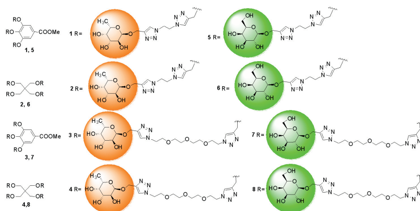
1. ábra. Multivalens fukozidok (1, 2, 3, 4) és galaktozidok (5, 6, 7, 8) szerkezete
