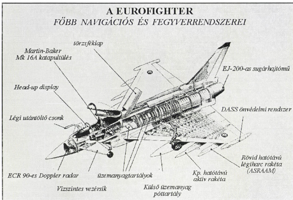
19. ábra: A Eurofighter főbb műszaki egységei
