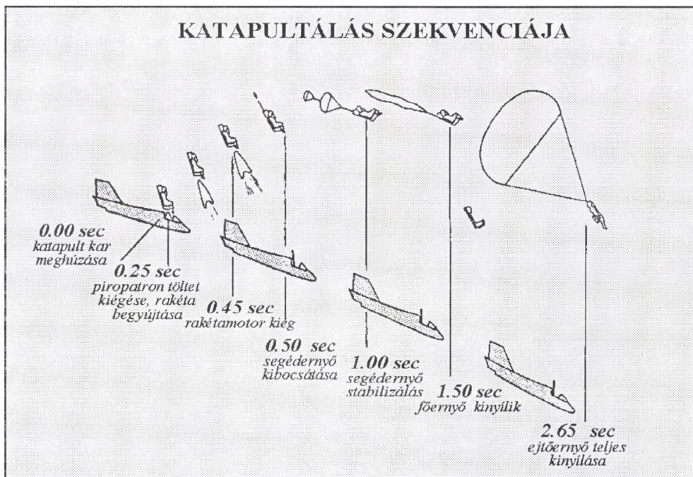
22. ábra: Katapultálás elvi vázlata
