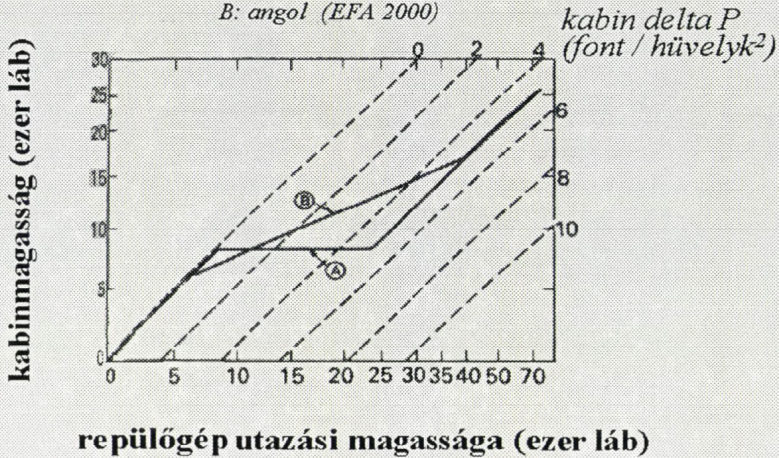
14. ábra: Az Eurofighter kabinnyomás profilja a magasság függvényében
