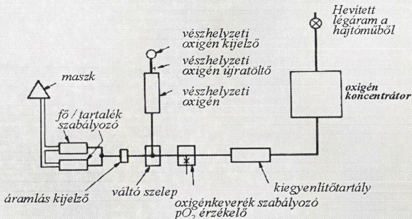
12. ábra: A fedélzeti oxigén rendszer vázlata
