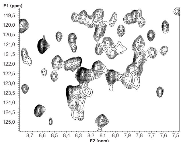
2. ábra. Egy ~20 kDa molekulatömegű rekombináns fehérje természetes izotóp-előfordulás mellett felvett ^1\text{H} - ^{15}\text{N} HSQC-spektruma. Minden egyes keresztcsúcs a spektrumban egy N-H-kötéshez rendelhető
