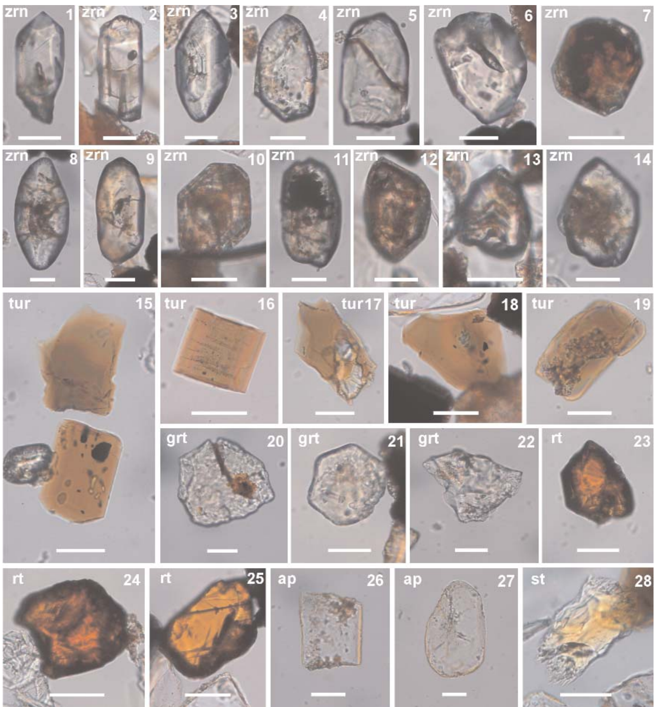
5. ábra. Nehézszárványok a Mecseknádasdi Homokkő Formáció felső-pliensbachi szakaszából, hibrid arenit, FA-64 minta (átesőfényes mikroszkópi képek, immerzió, n=1,66 ; a skála 50\ \mu\text{m} -nek felel meg)
