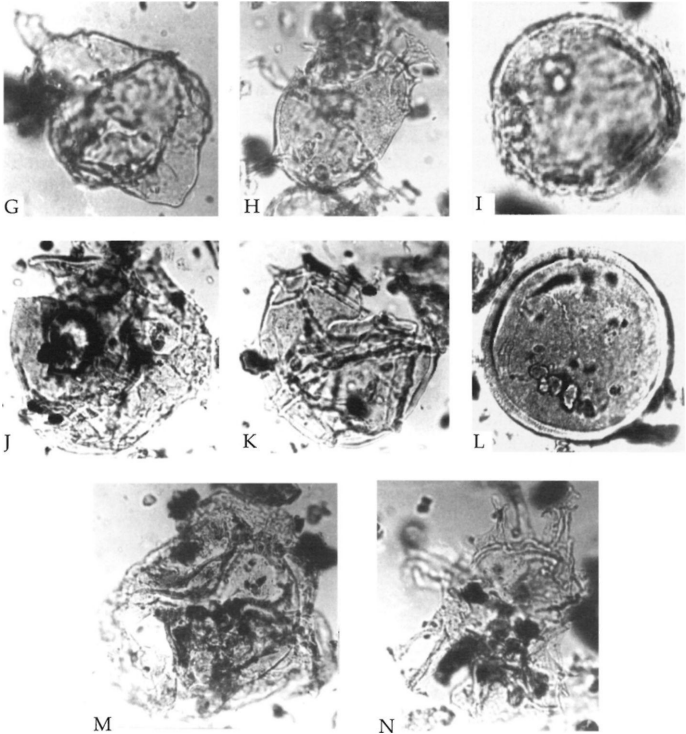
5. ábra. Szervesvázú mikroplankton a Battonya–pusztaföldvári-hátság fúrásaiból. G: Pontiadinium inequicornutum (BALTES 1971) STOVER & EVITT 1978, sima falú variáció, Battonya–K-8 fúrás 13. mag N.:650×; H: Spiniferites galeiformis SÜTŐ-SZENTAI 2000, Battonya–K-13 fúrás 6. mag N.:500×; I: Chytroeisphaeridia hungarica SÜTŐ-SZENTAI 1990, Battonya–K-8 fúrás 13. mag N.:750×; J: Spiniferites balcanicus (BALTES 1971) SÜTŐ-SZENTAI 2000, Battonya–K-8 fúrás 16. mag N.:550×; K: Millioudodinium pelagicum SÜTŐ-SZENTAI 1990, Battonya–K-8 fúrás 16. mag N.:530×; L: Tectatodinium pellitum WALL 1967, Battonya–K-8 fúrás 16. mag N.:470×; M: Galeacysta etrusca CORRADINI & BIFFI 1988, Battonya–K-13 fúrás 4. mag N.:390×; N: Spiniferites cruciformis WALL, DALE & HARADA 1973, Battonya–K-8 fúrás 9. mag N.:550×
