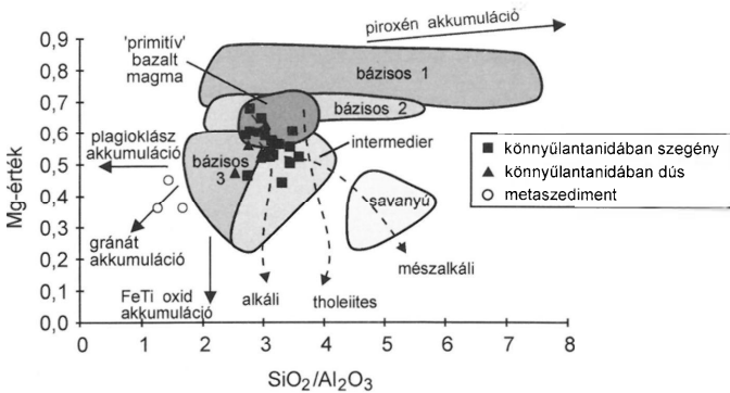
2. ábra. A granulit xenolitok összetétele az \text{SiO}_2/\text{Al}_2\text{O}_3 – Mg-érték diagramban. A különböző lelőhelyek bázisos, intermedier és savanyú alsókőreg xenolitjainak területe, valamint a „primitív” bazalt magma terület jelölése KEMPTON & HARMON (1992) alapján történt
