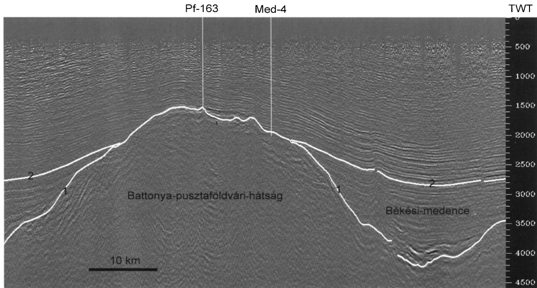
6. ábra. DNY-ÉK irányú szeizmikus szelvény a Battonya-pusztaföldvári-hátságon keresztül (nyomvonal az 1. ábrán). Jelmagyarázat: 1. neogén medence aljzata, 2. a Galeacysta etrusca zóna talpa a medencékben. A jelölt fúrásokban a mészmárga talpa idősebb, mint a Galeacysta etrusca zóna
