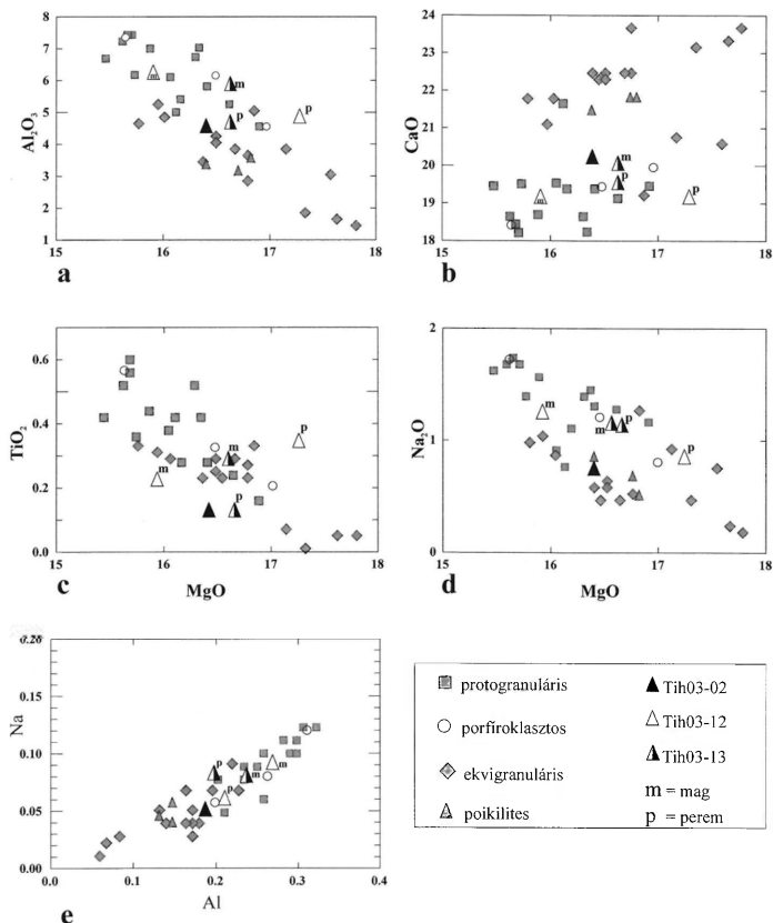
4. ábra. A vizsgált tihanyi kőzetzárványok klinopiroxénjeinek Al 2 O 3 -MgO (a); CaO-MgO (b); TiO 2 -MgO (c) valamint Na 2 O-MgO (d) Harker- (értékek m/m%-ban), illetve Al-Na diagramja (értékek kationszámban) (e) összehasonlításban a Bakony-Balaton-felvidék vulkáni terület más lelőhelyeinek összetételével. Összehasonlító adatok DOWNES et al. (1992), EMBEY-ISZTIN et al. (2001) és FALUS (2004) munkáinak felhasználásával
