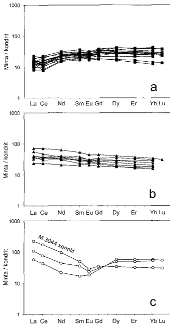
3. ábra. A Pannon-medence granulit xenolitjainak kondritnormált ritkaföldfém tartalma. A normálshoz használt kondrit összetétel PALME (1988) cikkéből származik. A jelölés a 2. ábra jelölésével azonos
