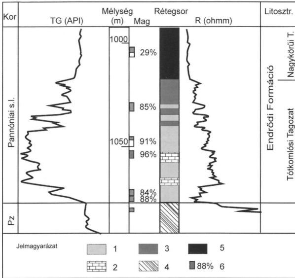
3. ábra. A Tótkomlósi Mészmarga Tagozat jellemző rétegsora egy battonyai fúrás példáján. Jelmagyarázat: 1. mészmarga, 2. mészkő, 3. márga, 4. metamorfit, 5. agyagmárga, 6. magminta, és a hozzá tartozó karbonáttartalom értéke
