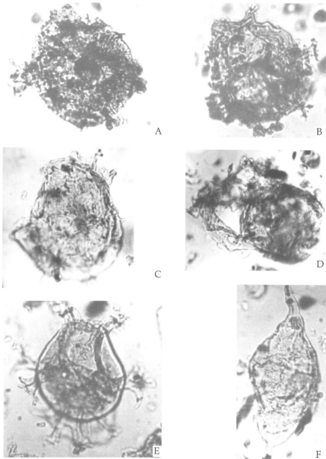
4. ábra. Szervesvázú mikroplankton a Battyonya–pusztaföldvári-hátság fúrásaiból. A-C: Spiniferites bentorii (ROSSIGNOL 1964) WALL & DALE 1970 pannonicus SÜTŐ-SZENTAI 1986, A: Mbh-1 fúrás 3 mag N.:610×; B,C: Kev-1 fúrás 1/3. mag N.:670×; D: Romanodinium areolatum BALTES 1971 új variáció, Battyonya K-8 fúrás 15/1. mag N.:660×; E: Spiniferites tihanyensis SÜTŐ-SZENTAI 2000, Battyonya K-8 fúrás 15/1 mag N.:700×; F: Pontiadinium inequicornutum (BALTES 1971) STOVER & EVITT 1978, Battyonya K-8 fúrás 15/1. mag N.:710×
