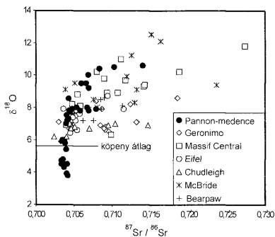
7. ábra. A Pannon-medence granulit xenolitjai \delta^{18}\text{O} és ^{87}\text{Sr}/^{86}\text{Sr} értékeinek összehasonlítása más területek granulit xenolitjeivel. Az összehasonlító adatok KEMPTON & HARMON (1992) munkájából származnak. Massif Central és Eifel (Európa), Geronimo és Bearpaw (É-Amerika), Chudleigh és McBride (Ausztrália)
