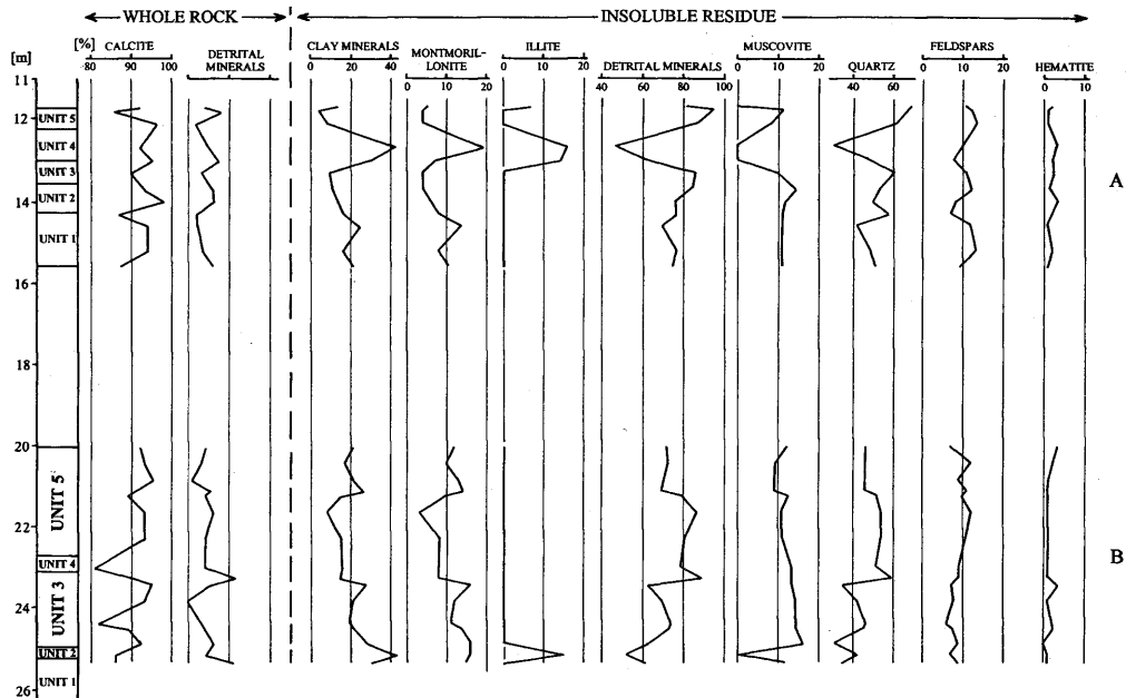
Fig. 15 Mineralogical composition of the travertine from Vértesszőlős
