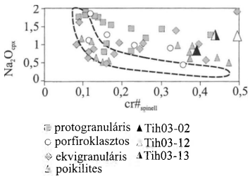
6. ábra. A vizsgált tihanyi kövezárványok klinopiroxénjeinek \text{Na}_2\text{O} -tartalma ( \text{Na}_2\text{O}_{\text{Cpx}} ) a spinellek \text{Cr} -értékéhez ( \text{Cr}^{\#}_{\text{spinel}} ) viszonyítva XU et al. (2003) alapján. A körbehatárolt terület a „normális” kimerülési trendet jelzi. Összehasonlító adatok DOWNES et al. (1992), EMBEY-ISZTIN et al. (2001) és FALUS (2004) munkáinak felhasználásával
