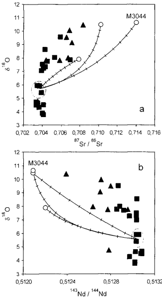
6. ábra. A Pannon-medence granulit xenolitjainak oxigénizotóp-arány és (a) ^{87}\text{Sr}/^{86}\text{Sr} , (b) ^{143}\text{Nd}/^{144}\text{Nd} diagramja a számított keverési hiperbolákkal. A bekerített terület a számítások során a köpeny szélsőkomponens becsléséhez használt xenolitokat mutatja. A jelölés a 2. ábra jelölésével azonos
