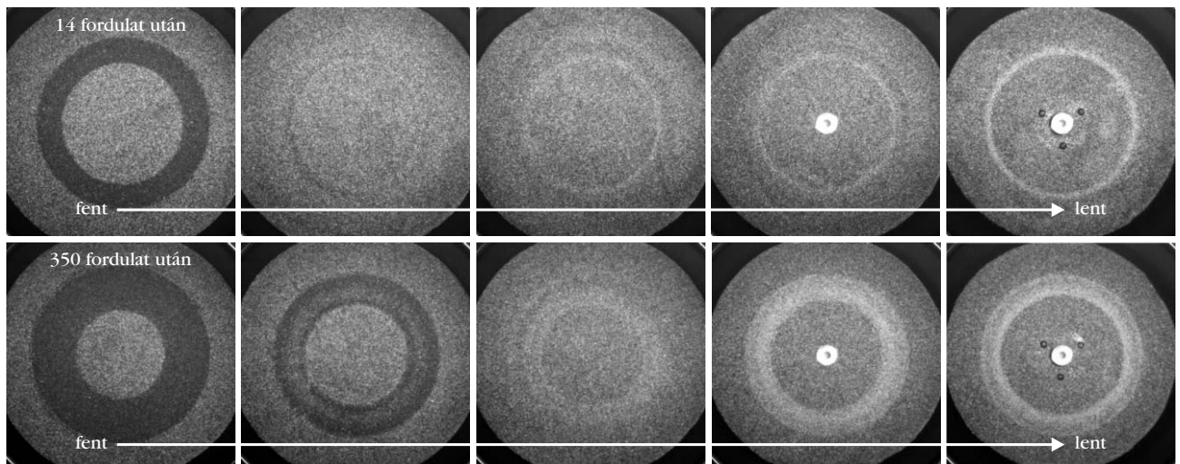
3. ábra. Szegregáció homok-üveggolyó keverékben. Felülnézeti képek a kísérlet végén elvégzett rétegenkénti feltárásról. A hengeres cellában a minta alatti tányér lassú forgatása következtében a nyírási zóna felszínén felhalmozódik a sötétebb színű homok, míg az üveggolyók a minta aljára vándorolnak. A henger átmérője 27 cm, a minta vastagsága 2 cm (50 részecskeátmérőnyi) volt.
