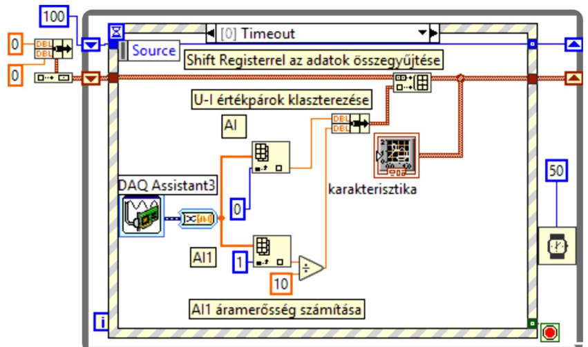
3. ábra. Az áramerősség (AI1) és a feszültség (AI0) egyidejű mérése a virtuális műszerben.
