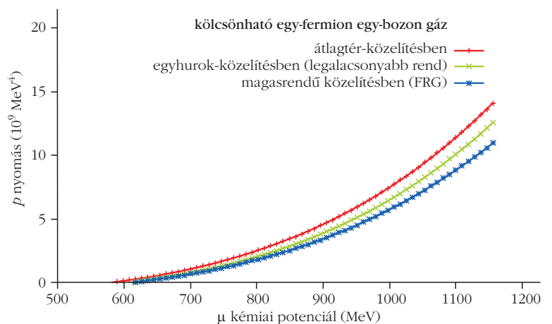
5. ábra. A kölcsönható egy-fermion egy-bozon gáz modell állapotegyenlete különböző közelítésekben számolva átlagtér, egyhuruk és az egzakt FRG esetben számolva.
