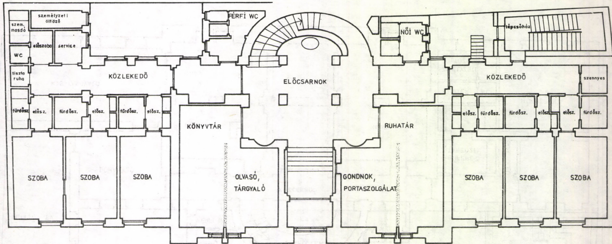
FÖLDSZINTI ALAPRAJZ
