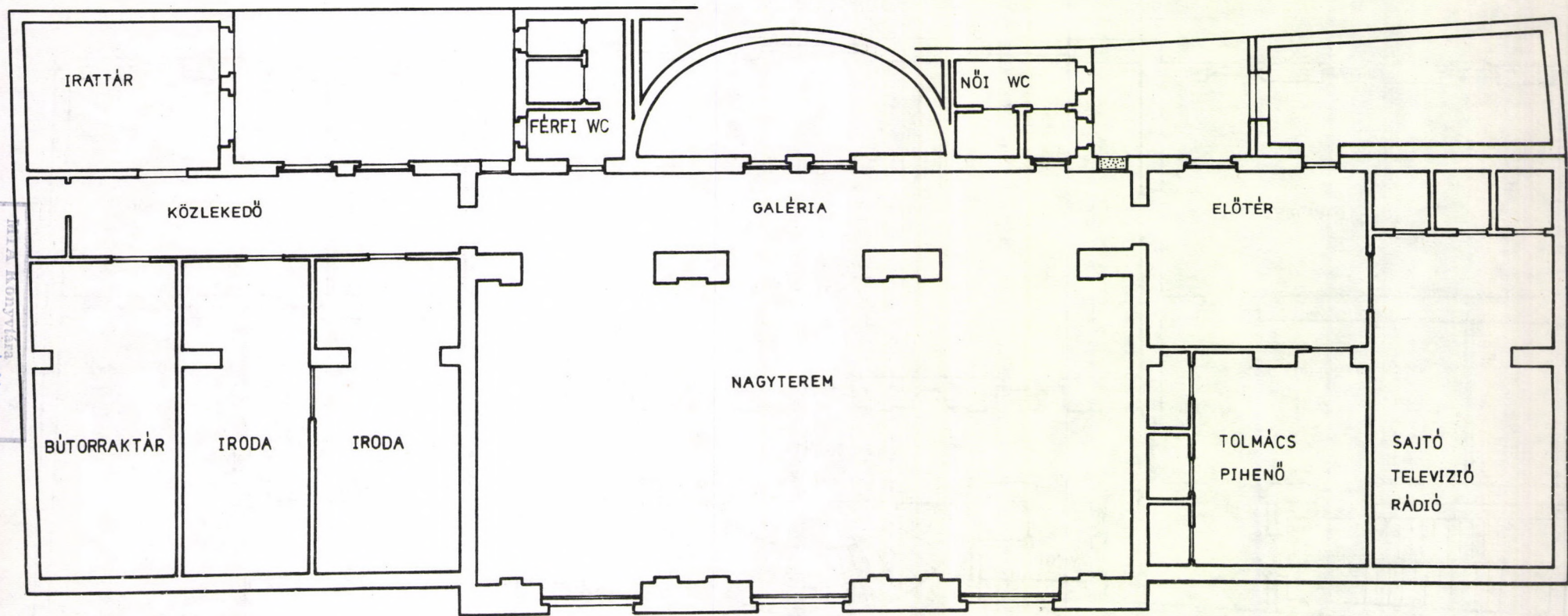
GALÉRIASZINT ALAPRAJZ
