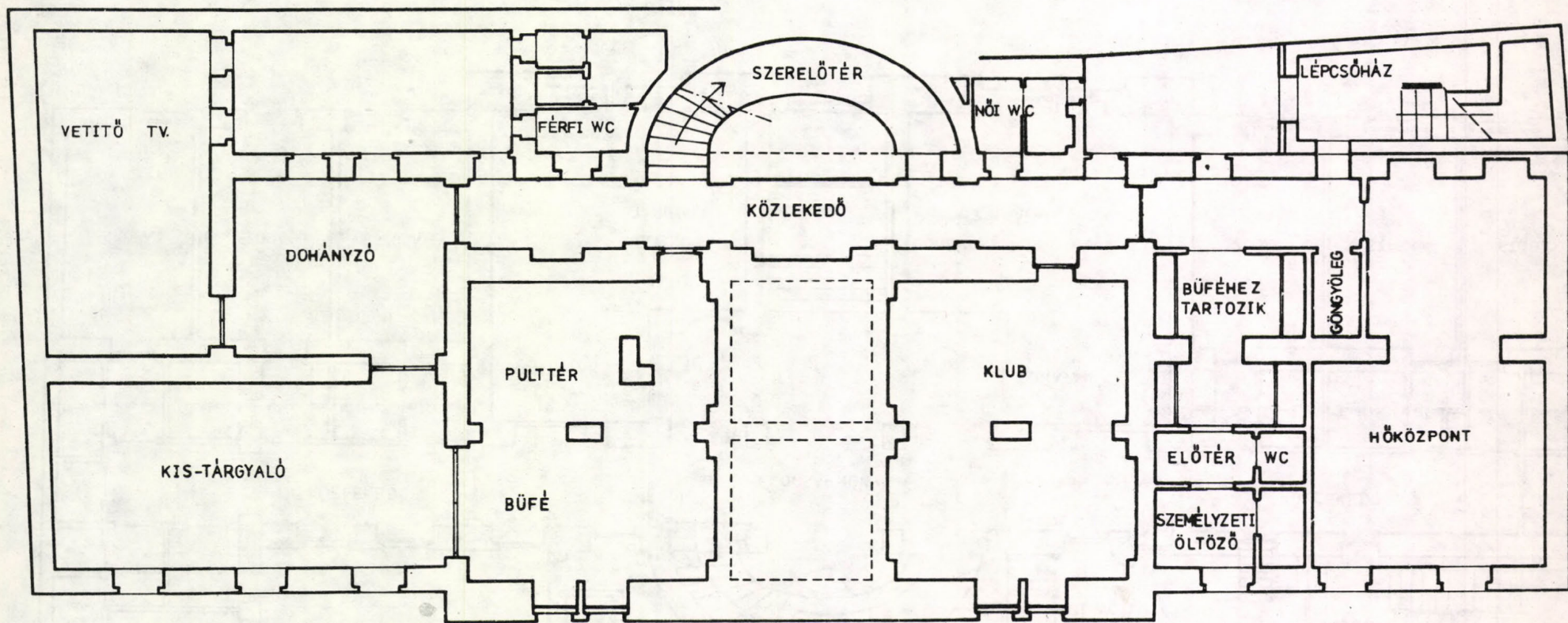
PINCE ALAPRAJZ
