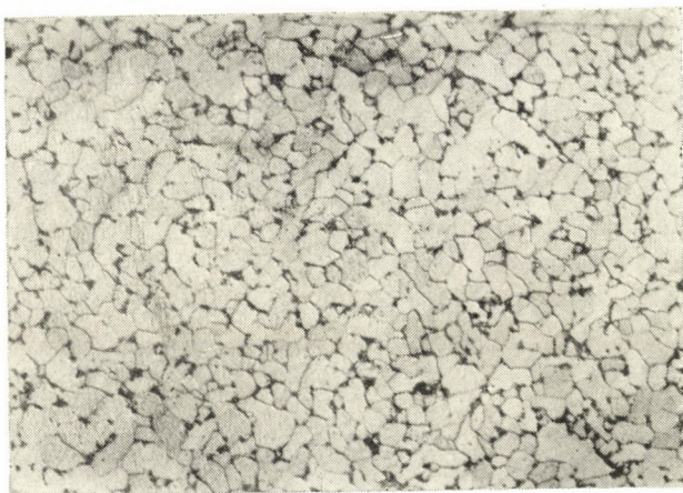
2. A zabla finom ferrites, kevés perlitet tartalmazó szövege. Maratás: nitál, N = 150 \times
