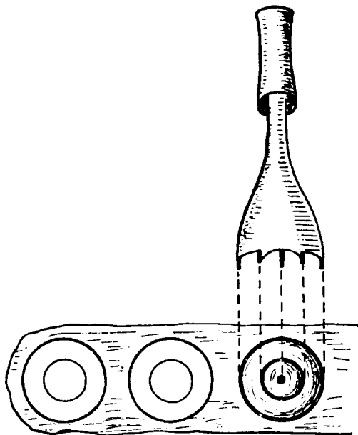
5. ábra. Az ötélú fúró rekonstrukciós rajza
