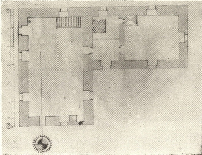
2. A hámori mellékműhely terve 1748-ból. OL Est. Lt. D. Léka 1748. nr. 1
