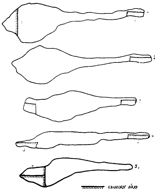
1. Megvizsgált honfoglaláskori nyílhegyek: 1, 2 jelű bodrogszerdahelyi, 3 jelű Szeged környéki, 4, 5 jelű Szabolcs megyei
