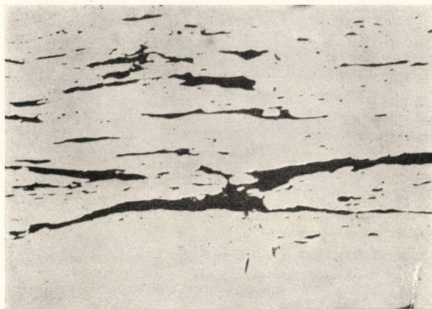
6. ábra. Salakzárványok maratlan hosszcsiszolaton. N = 100 \times
