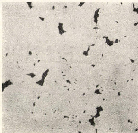
5. ábra. Salakzárványok maratlan keresztmetszeti csiszolaton. N = 100 \times
