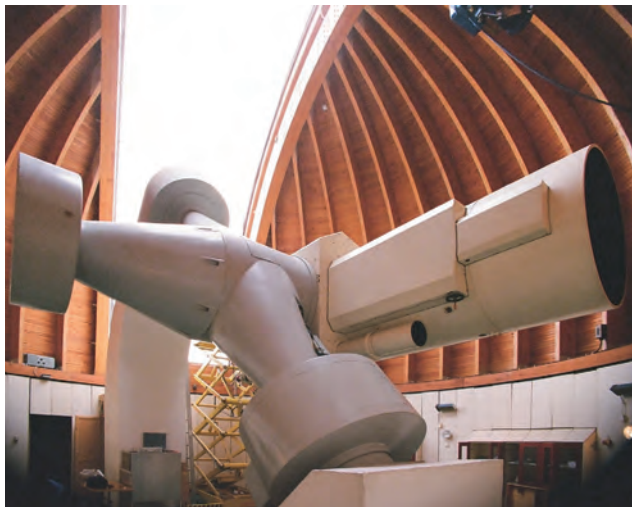
Az 1 méteres RCC teleszkóp Piskésetetőn (Fotó: Rácz Miklós)
