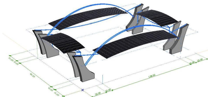
1. ábra. Szerkezeti tanulmány tangenciális feszített főtartóval gyámoltított szerkezetekre 2
