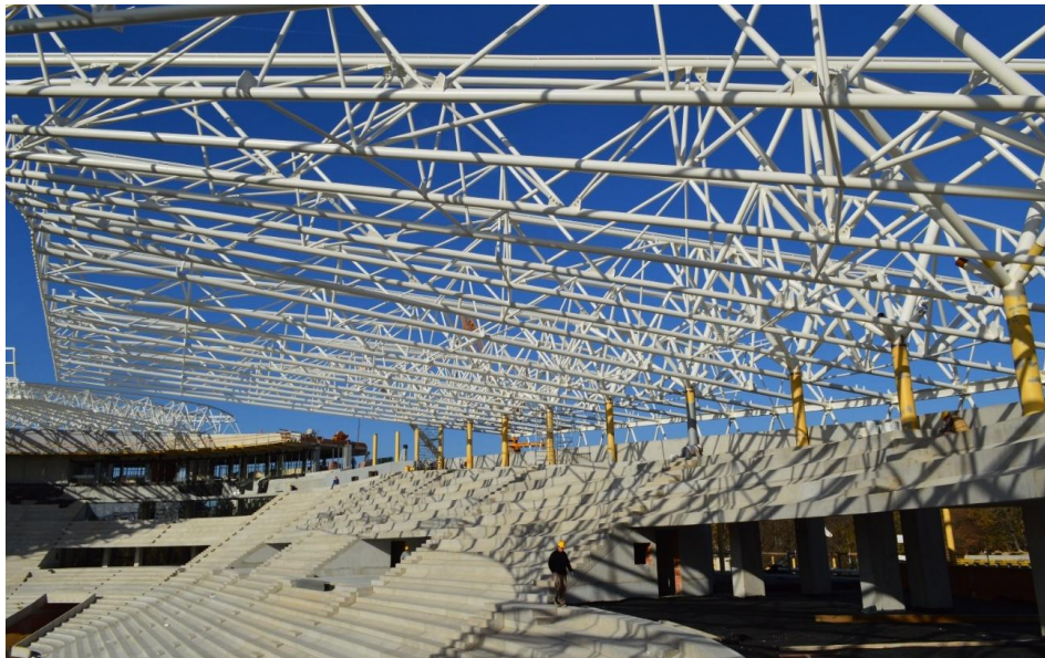
7. ábra. Rövidebb oldalak „átmeneti” tetőszerkezete szerelési állapotban
