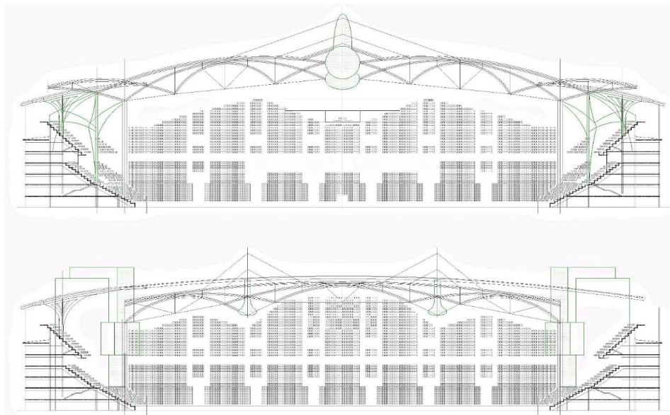
2. ábra. Szerkezeti tanulmány, „Főnix Aréna” tangenciális főtartós szerkezetre
