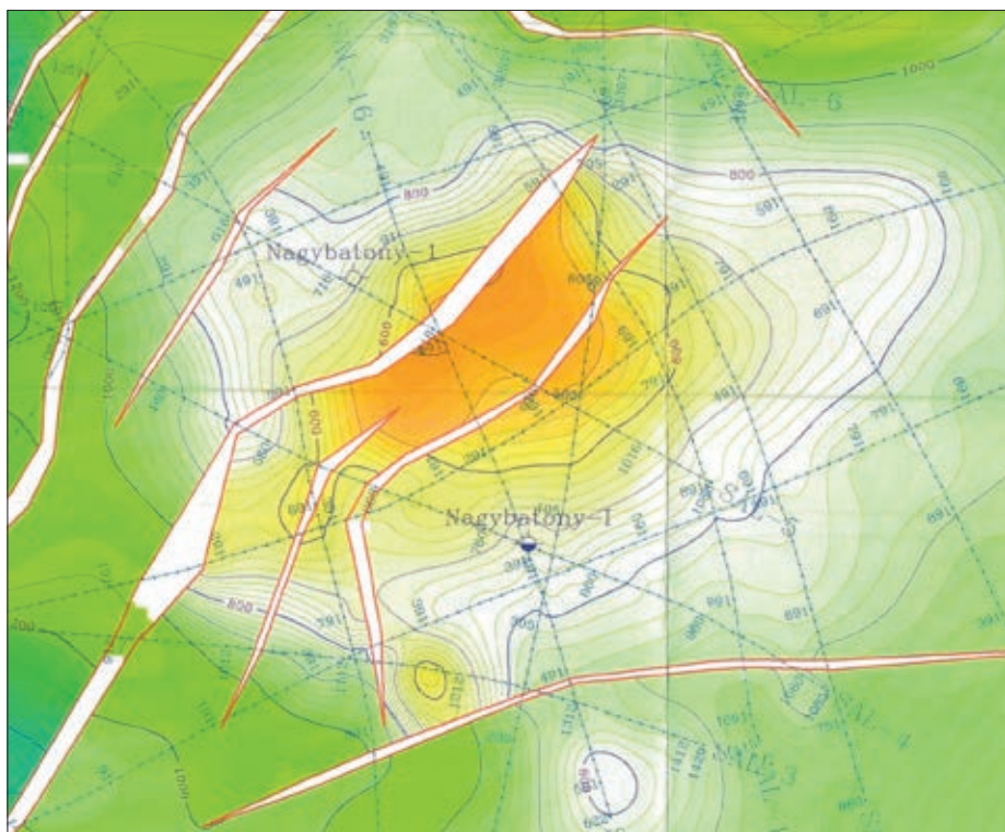
24. ábra: Az Alsólengyendi brachiantiklinális szerkezete az új mérések alapján (Nagybatony-1=Nb-324, az oligocén fekü szeizmikus időtérképe, vonatkozási szint +50 m, Boncz L.-Sóreg V. 2012. 7. mell).
