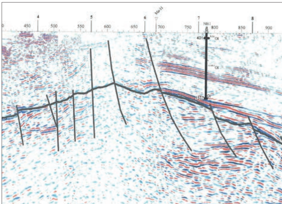
23. ábra: SAL-4 szeizmikus szelvényen látható antiklinális szerkezet az Nb-I. fúrással (a fúrás az Egyház magasán van, Kiss J. et al. 2011).
