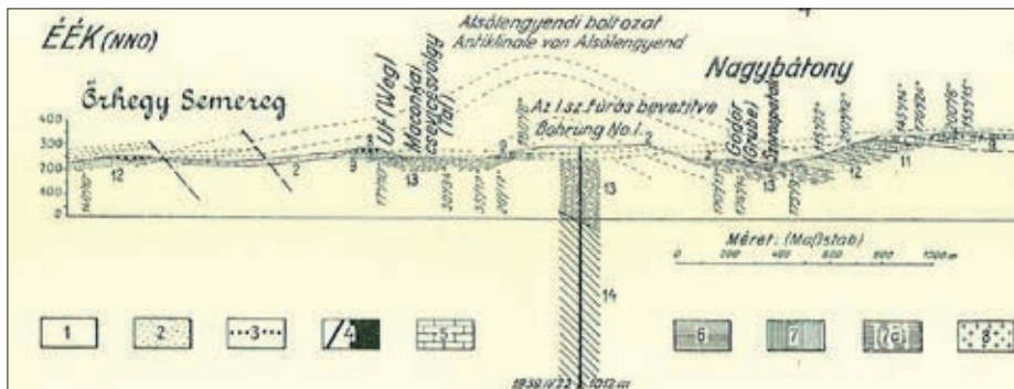
10. ábra. Földtani szelvény az antiklinálison keresztül, amin túlságosan hangsúlyosan jelölik a boltozatot (Schréter Z. 1940b. 4. szelvény).
