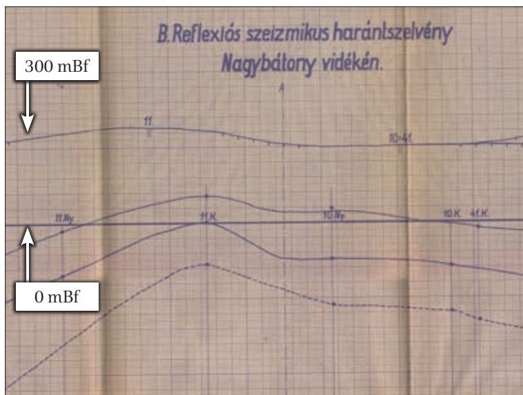
8. ábra: Ny-K-i irányú szeizmikus reflexiós szelvény az Egyház magasa alatti „búbbal” (Bassó I. 1938. melléklet részlete).
