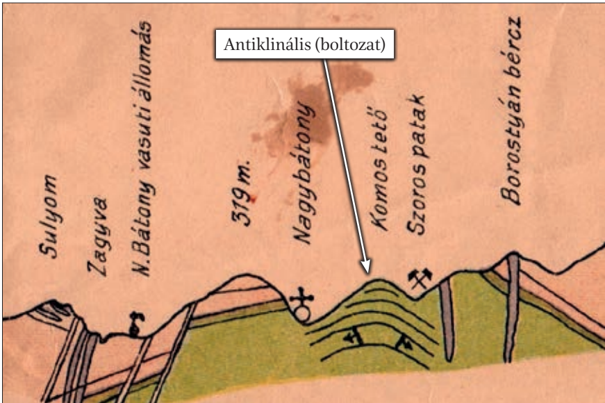
3. ábra: A nagybátonyi antiklinális földtani szelvénye, vertikális szerkezete (id. Noszky J. 1926. térképén lévő szelvényről, részlet).
