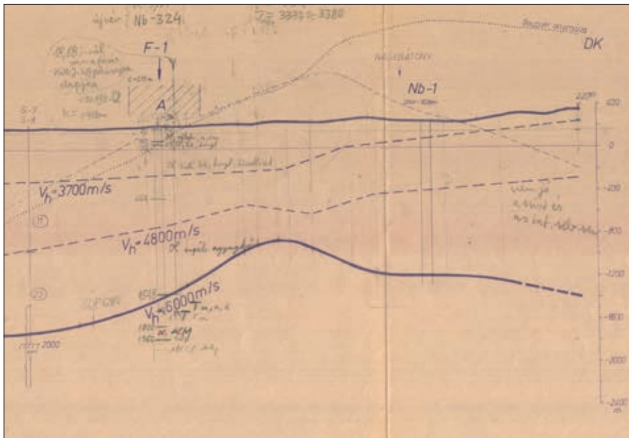
22. ábra: A Sá-1 ÉNy-DK-i irányú szeizmikus szelvény részlete. Az alaphegységi boltozat tetőpontja ÉNy-i irányba helyezkedik el a Nb-I. fúrástól, éppen a Tóberke irányába (Hobot J.-Szabadvány F. 1970. 8. mell).
