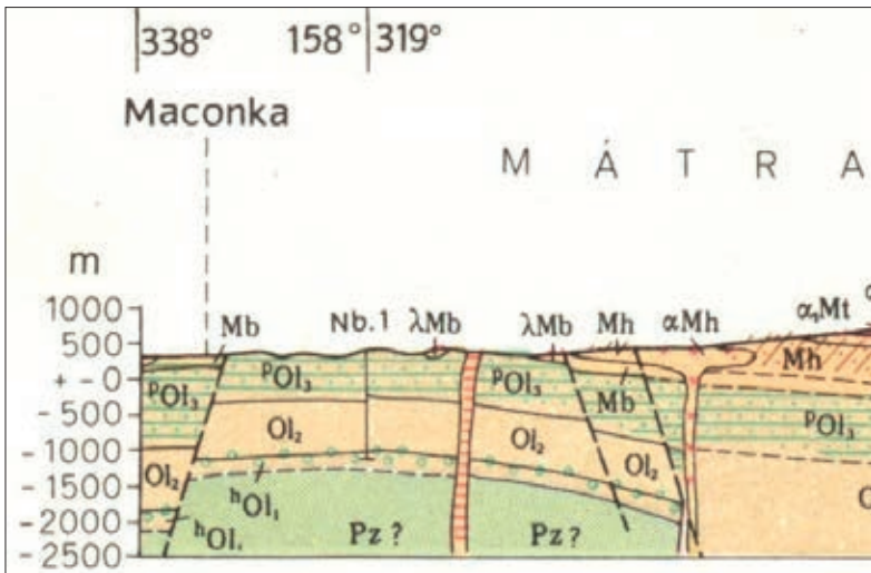
20. ábra: ÉÉNy-DDK-i irányú szelvény az antiklinálison keresztül, benne az Nb-I. kincstári fúrás által harántolt rétegekkel: hOl1=Hárshegyi homokkő, halpikkelyes- és tűzálló agyag, Ol2=Foraminiferás agyagmárga, pOl3=Pectunculuszos agyagmárga (Jámbor Á. et al. 1966).
