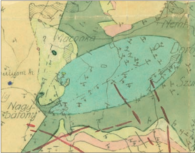
4. ábra: Az Alsólengyendi brachiantiklinális térképe (horizontális kiterjedése) a dőlés-csapás mérések alapján (Schréter Z. én, részlet).
