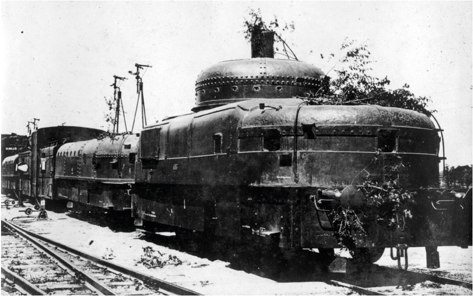
3. kép: Az Osztrák–Magyar Monarchia „lapos” szerelvénye és annak önjáró lövegkocsija 1916. (Fortepan, 52263)
