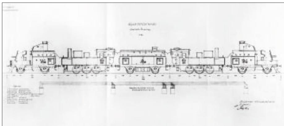
2. kép: Az Osztrák–Magyar Monarchia nehéz páncélvonatainak műszaki rajza 1915. (MMKMA RA-581: Páncélvonat Északi Főműhely)
