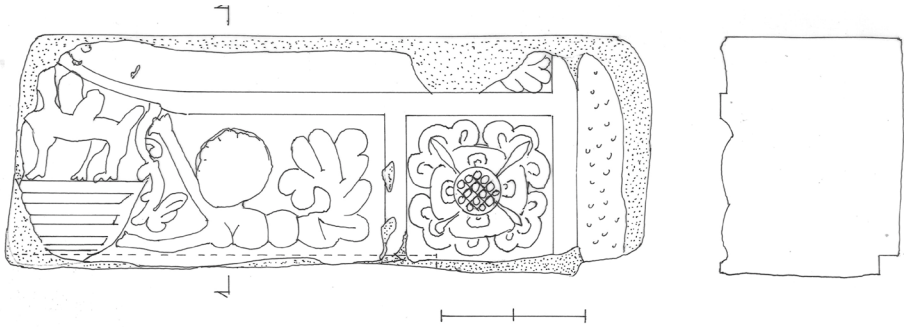
4. kép: Címeres szemöldökkő felmérési rajza
