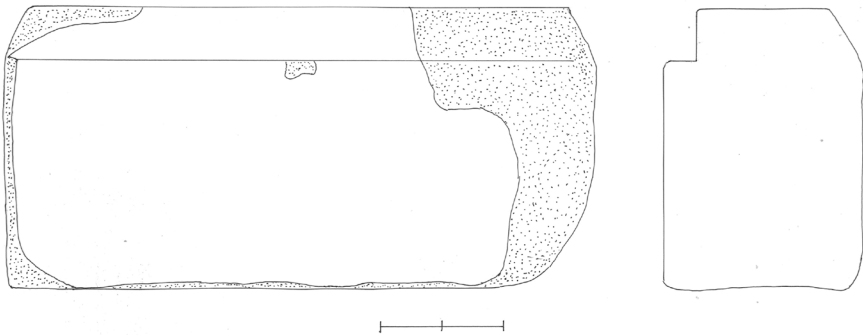
2. kép: Keretkő felmérési rajza
